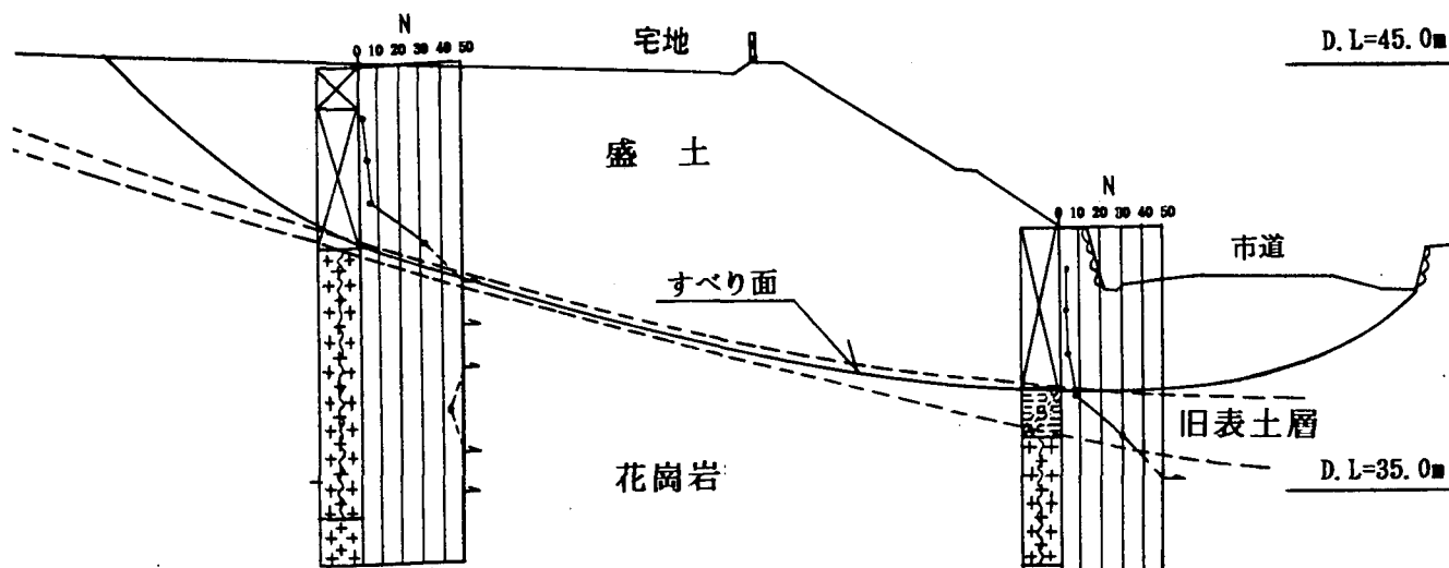
図-3 検討断面〔文献2〕に加筆
