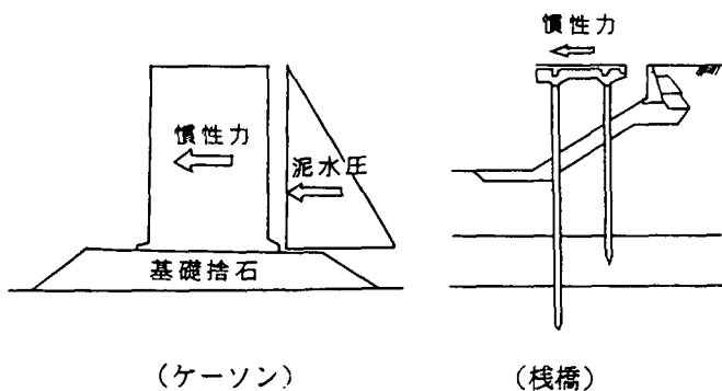
図 3 荷重条件
