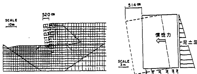
図6 ケーソン変形図
