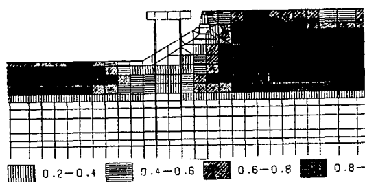
図5 栈橋の過剰間隙水圧比分布
