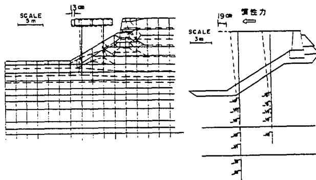
図7 栈橋変形図
