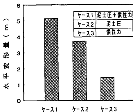
図8 各外力と水平変形量の関係
