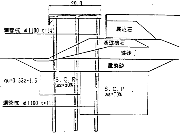
図10 栈橋の標準断面
