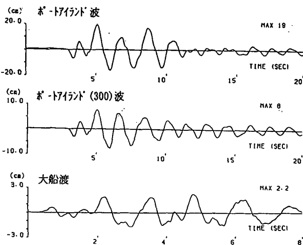
図一8 杭頭での変位時刻歴図 (一次元モデル: 非線形)
