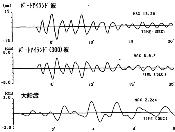
図一6 杭頭での変位時刻歴図 (二次元モデル)
