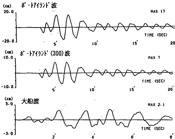
図一7 杭頭での変位時刻歴図 (一次元モデル: 線形)
