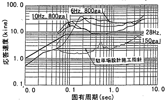
図-3 速度応答スペクトルの比較
