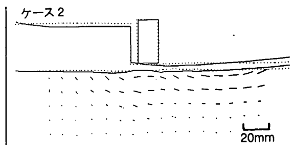
図3 残留変位ベクトル(シリーズ1)
