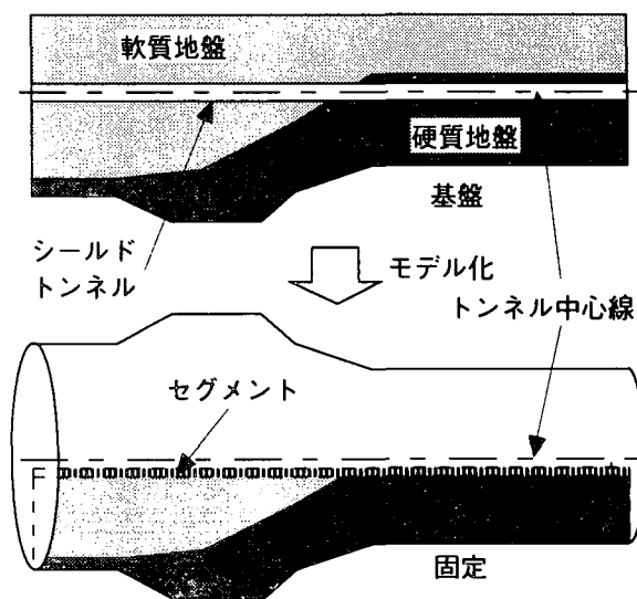
図-1 軸対称モデルの概念図
