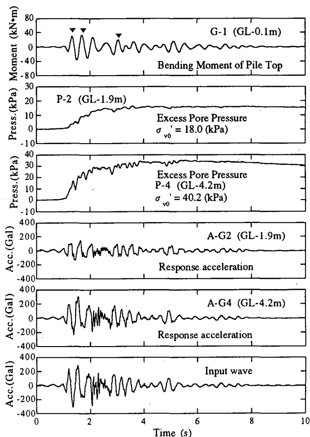
(b) 遠心振動実験
