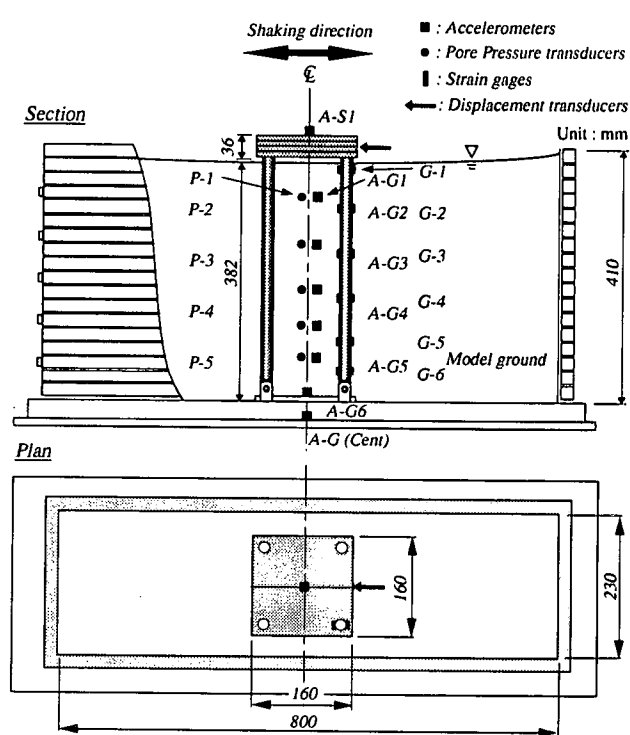
図-3 遠心振動実験の計器配置
