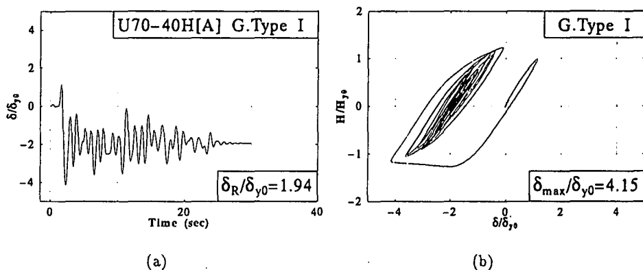
Fig.4 ハイブリッド実験結果 (地震波：土木研究所レベル 2，地盤種 I)
