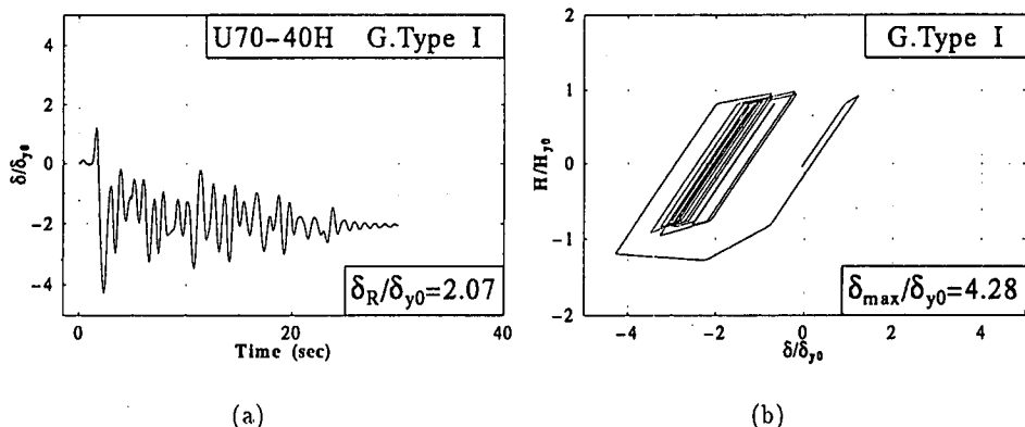
Fig.5 応答解析結果 (地震波：土木研究所レベル2，地盤種Ⅰ)
