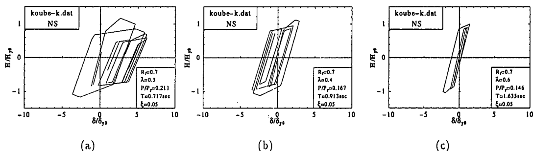
Fig.7 応答解析結果-復元カールプ (地震波：神戸海洋気象台，NS 成分)
