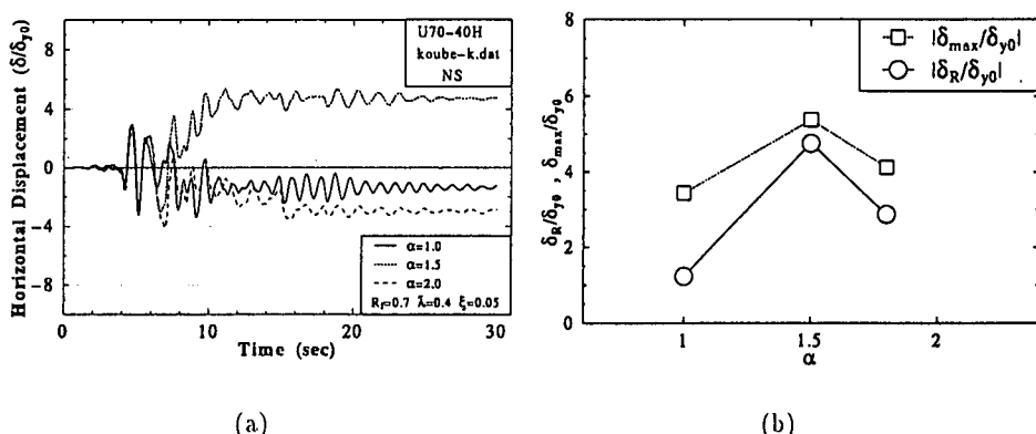
Fig.8 鉛直地震動を考慮した応答解析 (地震波：神戸海洋気象台，NS 成分)
