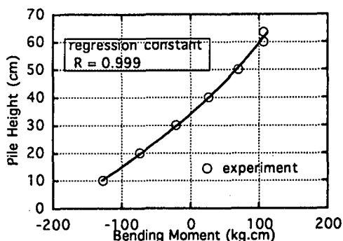
図6 杭体外力による曲げモーメント (ケース1)
