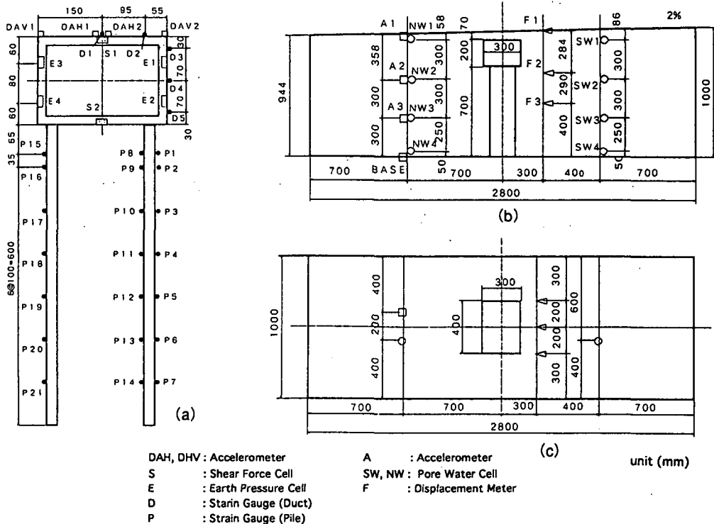
図1 計測点配置 (a) 洞道・杭, (b) 地盤 (平面), (c) 地盤 (側面)
