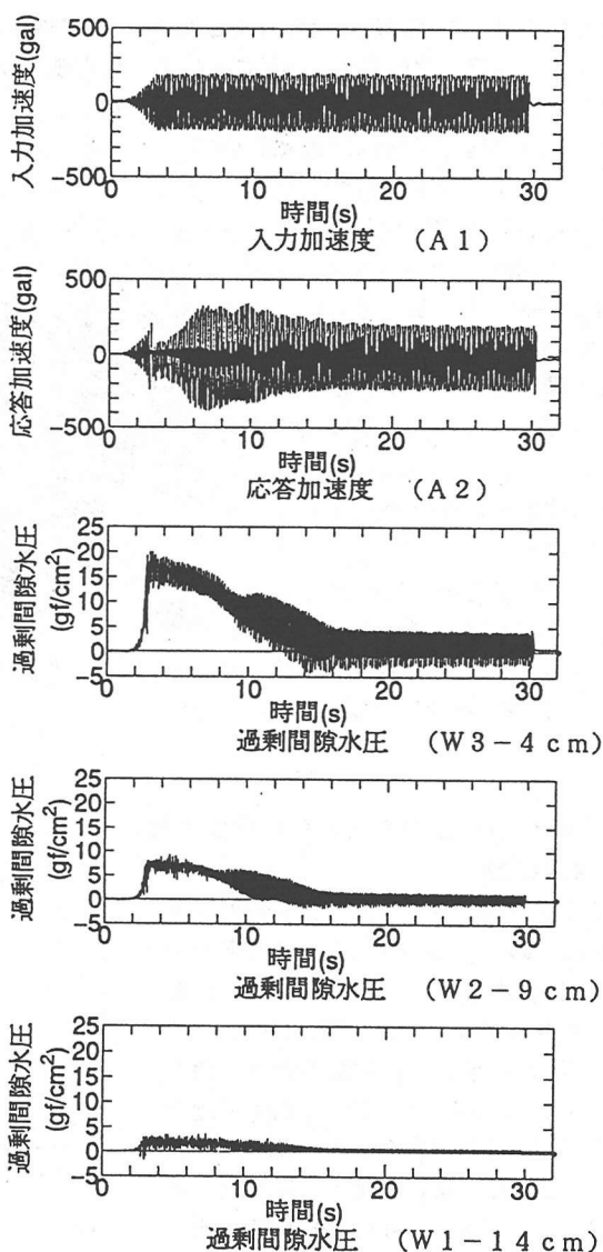
図2 波形の時刻歴の一例 (混合率50%, 入力加速度230gal)
