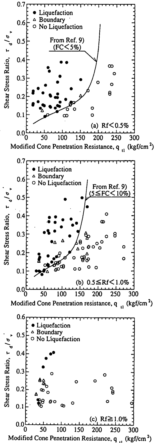
図-5 摩擦比で分けた液状化強度と換算先端抵抗の関係
