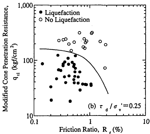
図-4 摩擦比で分けた換算先端抵抗と摩擦比の関係
