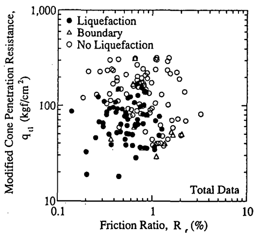
図-3 換算先端抵抗と摩擦比の関係
