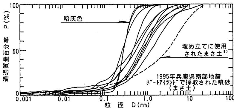
図-5 ポートアイランドで生じた噴砂の粒度組成
