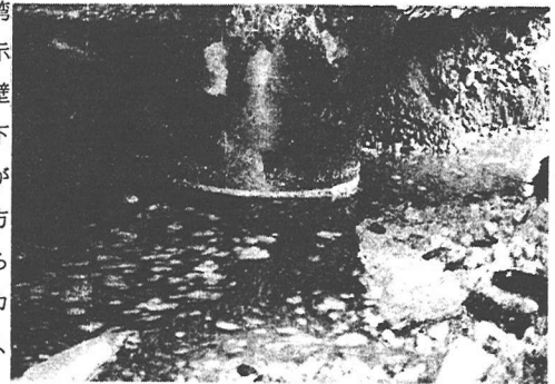
写真-2 中央市場魚バ場基礎杭の被害
