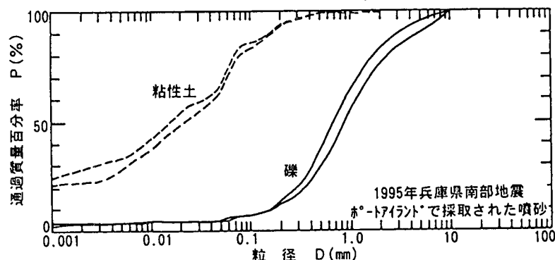
図-7 噴砂丘周辺の粘性土と噴砂丘の粒度組成
