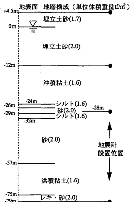
図-1 神戸ポートアイランドにおけるアレー観測地点位置図、および想定した地層構成
