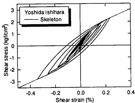
図-5 第3層の応力-ひずみ関係
