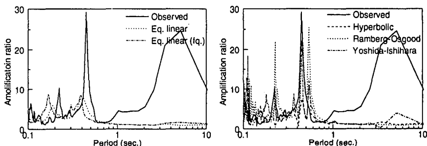
図-6 周波数増幅関数
