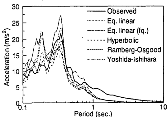
図-7 応答スペクトル
