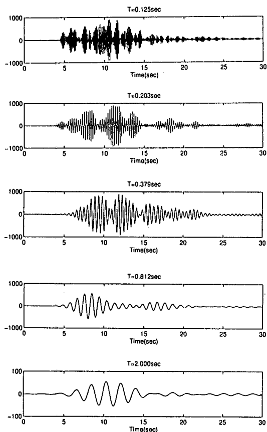
図5 各成分別に再構成した波形
