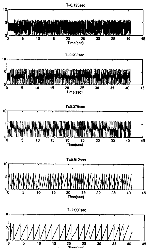
図7 位相の時間変動
