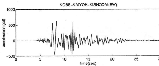
図1 兵庫県南部地震・神戸海洋気象台における加速度記録 (EW成分)
