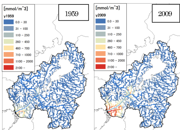
図-8 1959年，2009年における底質の水銀濃度分分布比較
