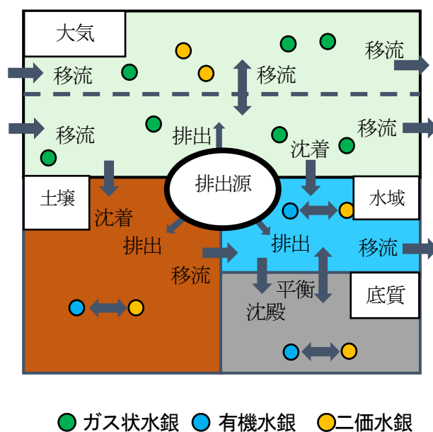
図-1 多媒体モデルの概要図
