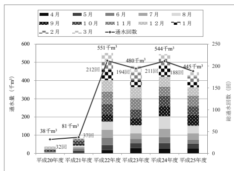
図-7 通水量と通水回数
