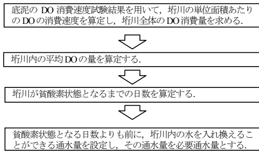
図-9 必要導水量の設定方法
