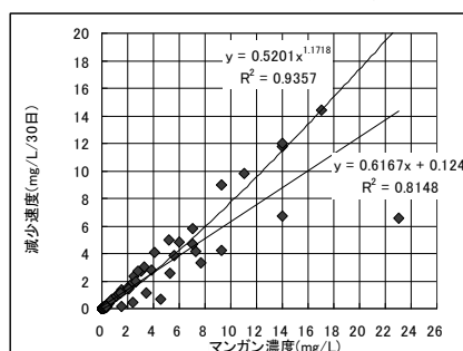
図-14 マンガンの減少速度
