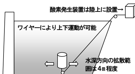
図-4 高濃度酸素溶解装置の特徴
