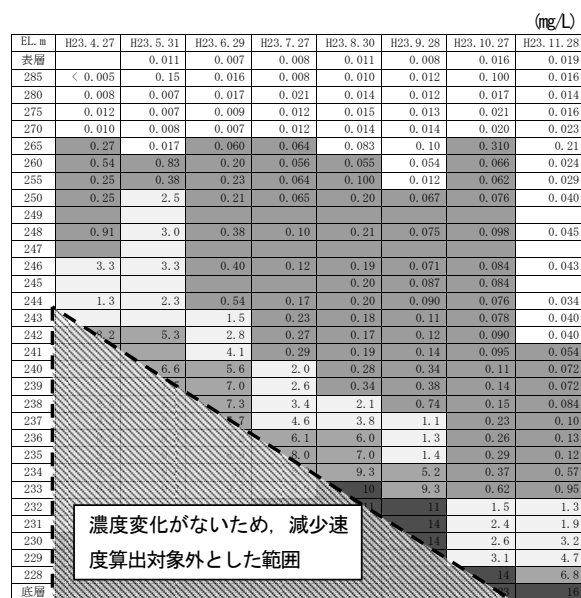
図-13 全マンガン濃度の経月変化
