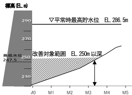
図-5 改善対象範囲（縦断面図）
