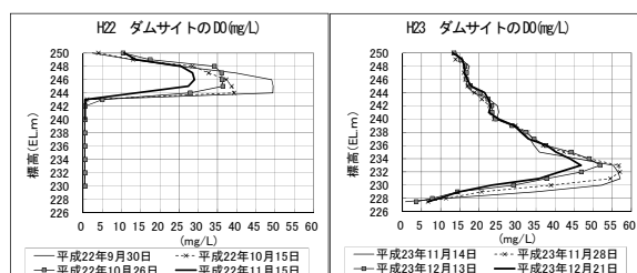
図-12 装置停止時のDO変化
