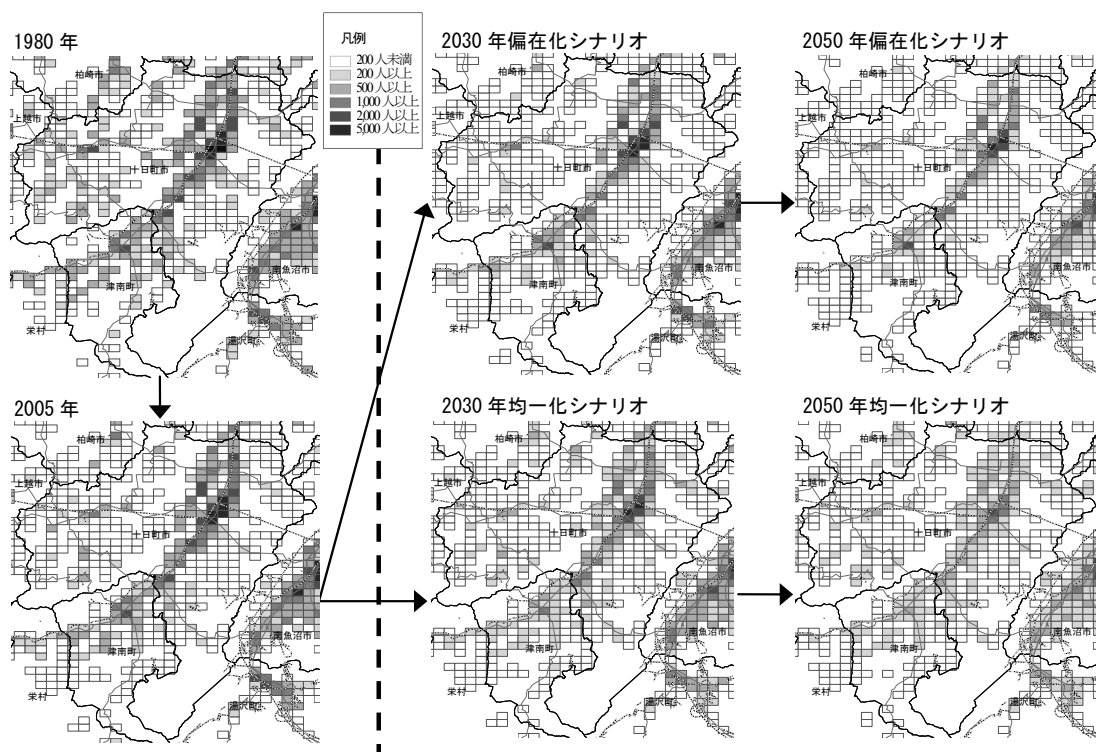
図-4 シナリオ別人口分布の変化（新潟県十日町市）
