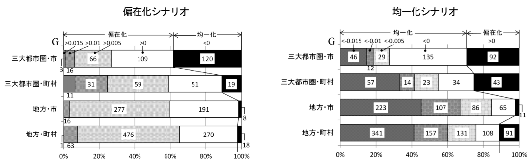
図-7 2005→50年の人口分布ジニ係数の全国的な変化
