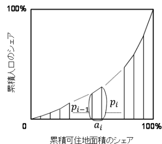
図-2 人口分布ジニ係数の定義
