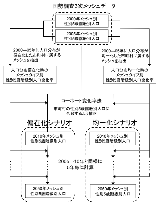
図-1 偏在化・均一化シナリオ構築のフロー
