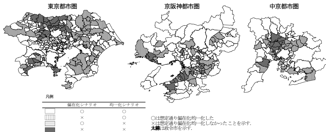
図-8 三大都市圏の市町村におけるシナリオ想定への適合・不適合
