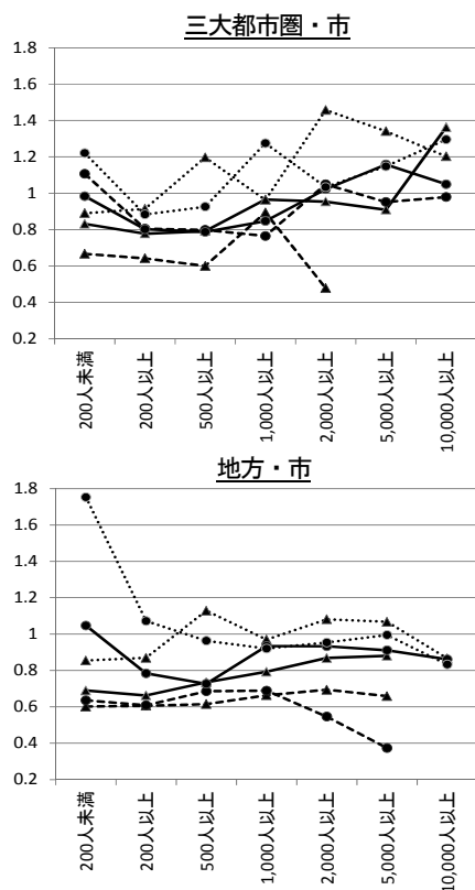
図-3 人口変化率（男性15～19歳→20～24歳の例）（縦軸は人口変化率、横軸はメッシュ人口規模を示す）
