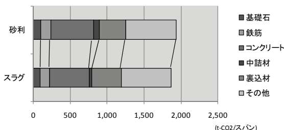
図-6 資材別の二酸化炭素排出量
