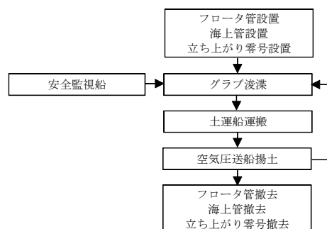
図-8 浚渫工事の施工手順
