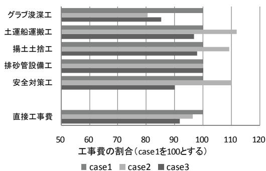
図-12 工種毎の工事費の割合比較
