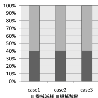
図-11 項目別の二酸化炭素排出割合
