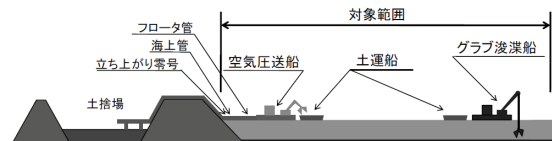
図-9 浚渫工事のイメージ
