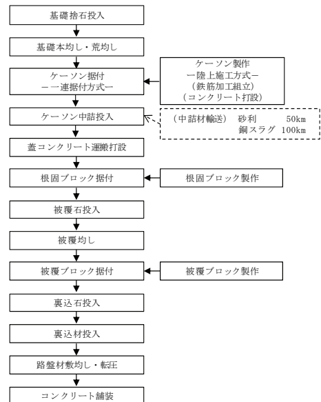
図-3 ケーソン式係船岸の施工手順
