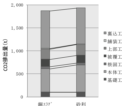
図-4 工種別の二酸化炭素排出量
