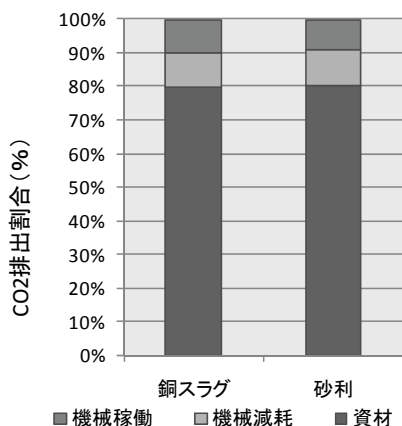
図-5 項目別の二酸化炭素排出割合
