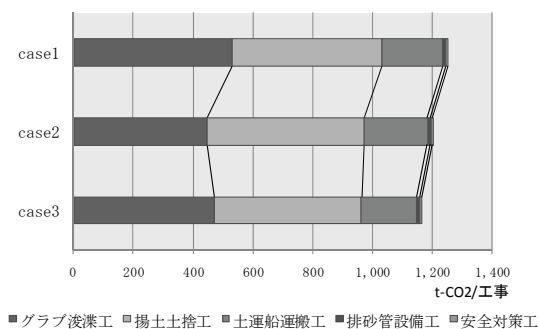
図-10 工種別の二酸化炭素排出量
