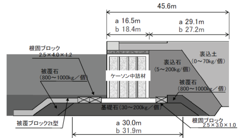
図-2 ケーソン式係船岸断面図
