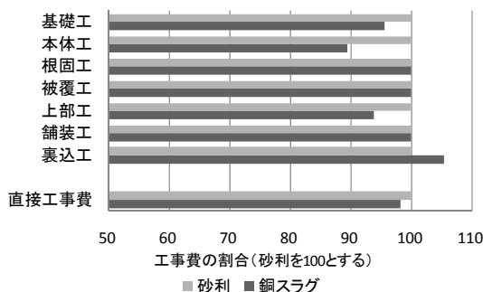
図-7 工種毎の工事費割合比較
