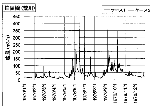
図-13 笹目橋（荒川）地点における流量比較
