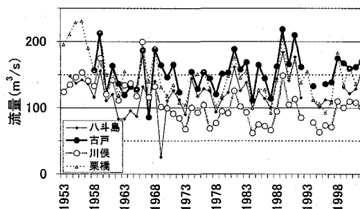
図-11 利根川における利根大堰を挟む各地点の平水流量の経年変化
