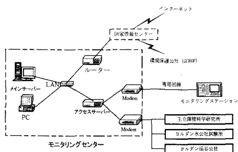
図-3 テレメトリシステムの全体概要
