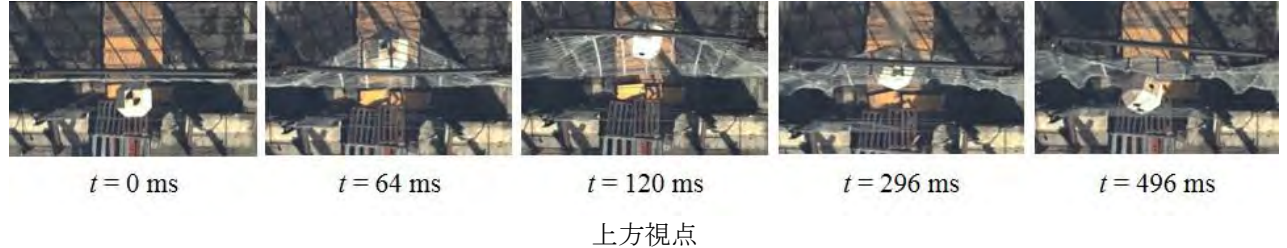
写真-5 H-7 試験体の変形状況
