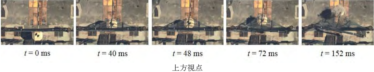
写真-4 C-5 試験体の変形状況
