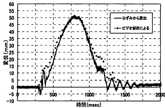
図-8 変位～時間関係
