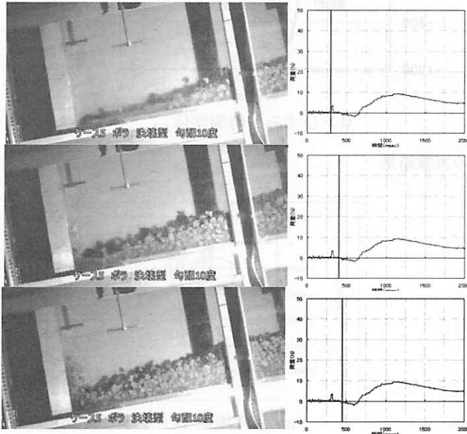
(a) くさび形状を示す場合 (No.5)
