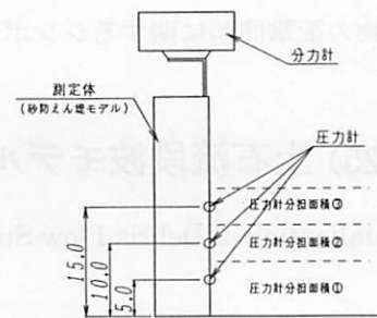
図-3 荷重測定
