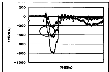
(b) 固有周期 T=0.2sec(No.18)
