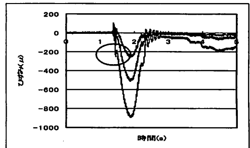
(a) 固有周期 T=0.1sec(No.15)
