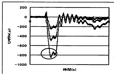
(c) 固有周期 T=0.3sec(No.21)
