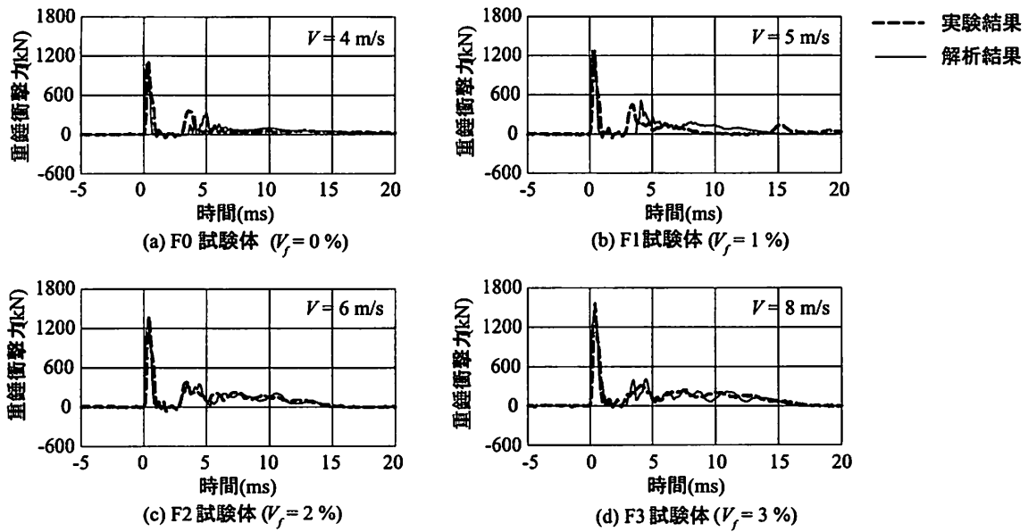
図-7 重錘衝撃力波形に関する実験および数値解析結果の比較図
