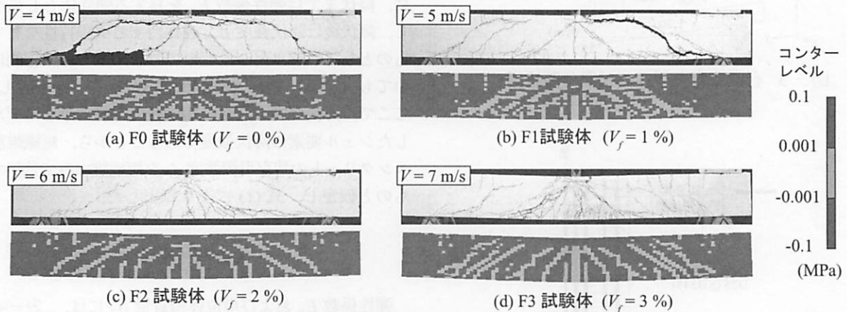
図-6 ひび割れ分布性状に関する実験および解析結果の比較
