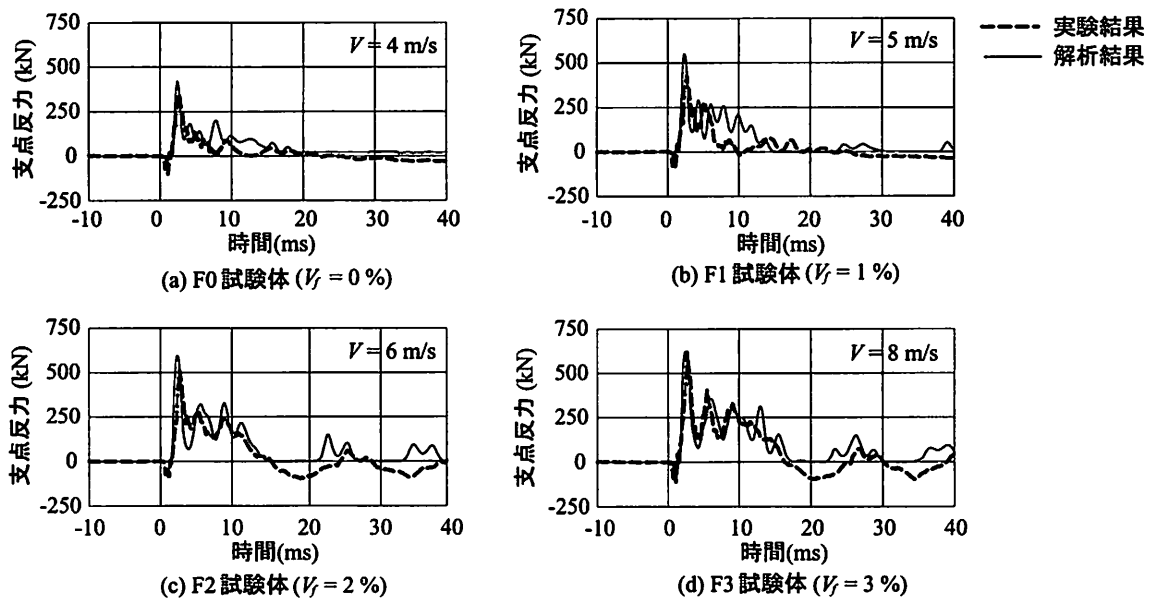
図-8 支点反力波形に関する実験および数値解析結果の比較図
