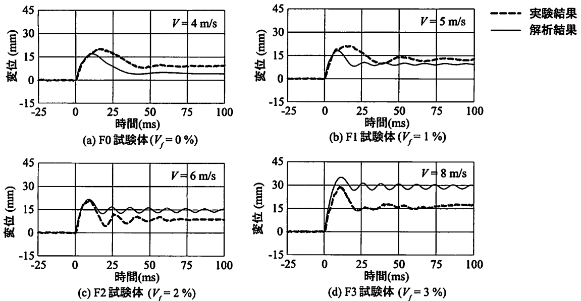
図-9 変位波形に関する実験および数値解析結果の比較図
