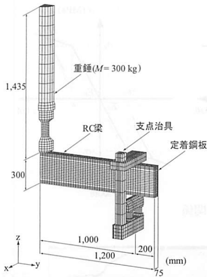
図-3 有限要素モデルの要素分割状況
