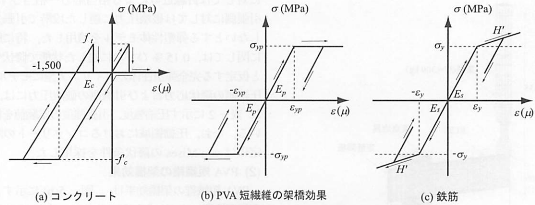
図-5 各材料の応力-ひずみ関係
