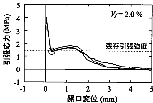
図-2 短繊維混入コンクリートの引張応力-開口変位関係の一例 5)
