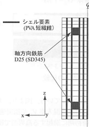
図-4 有限要素モデルにおけるRC梁の断面図
