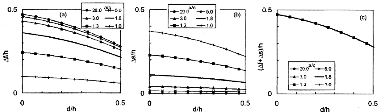
図-4 掘削幅直径比とマンホール高さ h で正規化した地下水位深さと(a)最大浮上がり量、(b)沈下量、(c)鉛直変位量の関係
