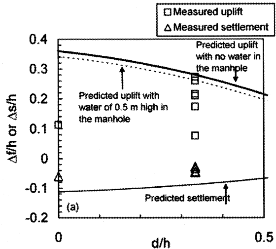
図-12 実験結果と提案法により予測される最大浮上がり量と最大沈下量: 浸水によるマンホール重量の増加を考慮した場合を点線で示す
