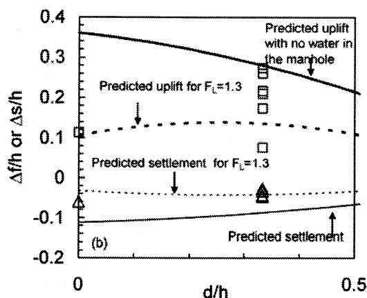
図-14 実験結果と提案法により予測される最大浮上がり量と最大沈下量：液状化安全率 ( F_L ) を1.3とした場合の曲線を点線で示す。
