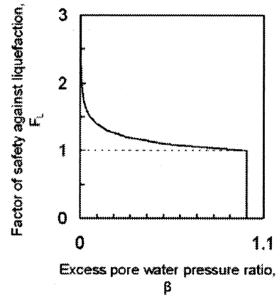
図-5 液状化安全率 ( F_L ) と過剰間隙水圧比 ( \beta ) の関係 11)
