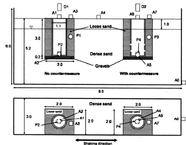
図-7 遠心模型とセンサーの設置位置 (単位はm)
