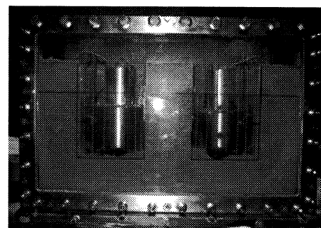
図-8 マンホール模型設置後、埋戻し前の状況
