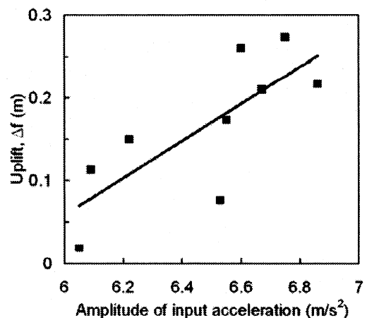
図-13 入力加速度振幅最大値と浮上量
