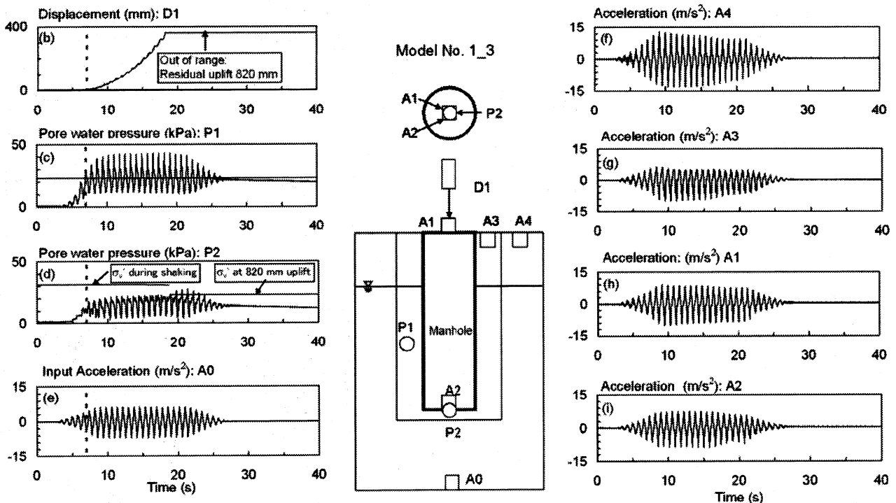
図-10 実験ケース5における計測値
