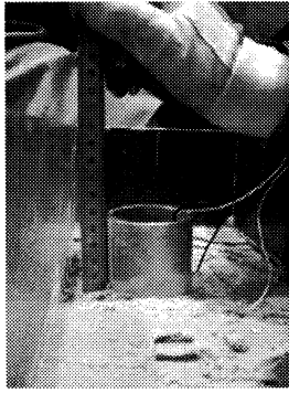
図-11 加振後のマンホール(ケース5)
