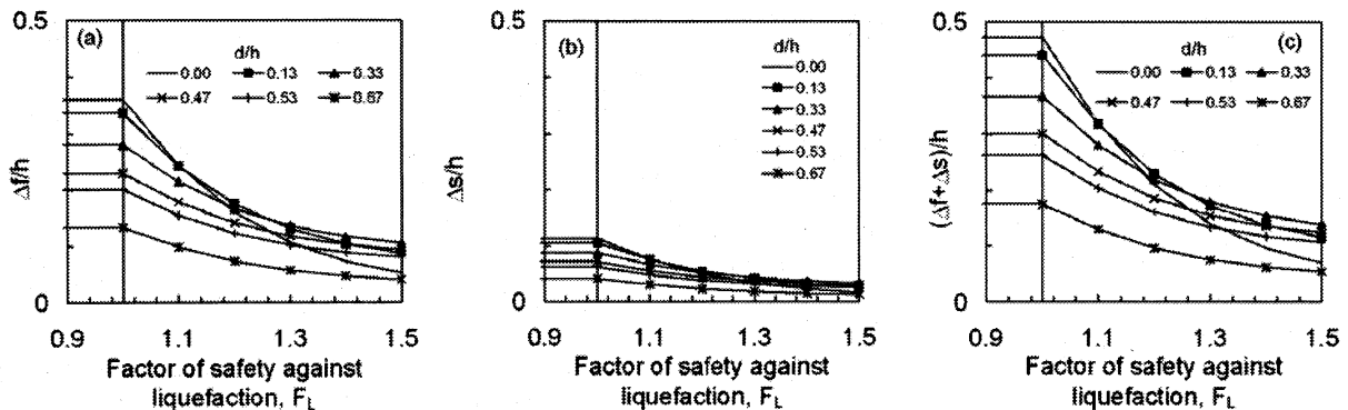
図-6 液状化安全率とマンホール高さ h で正規化した(a)浮上がり量、(b)沈下量、(c)鉛直変位量
