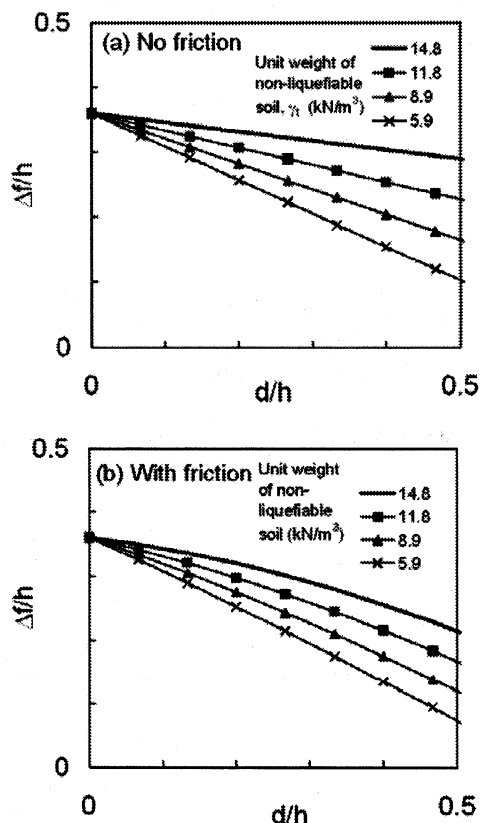
図-3 マンホール高さ h で正規化した地下水位深さと最大浮上がり量との関係：(a)周面摩擦を考慮しない場合、(b)周面摩擦を考慮した場合
