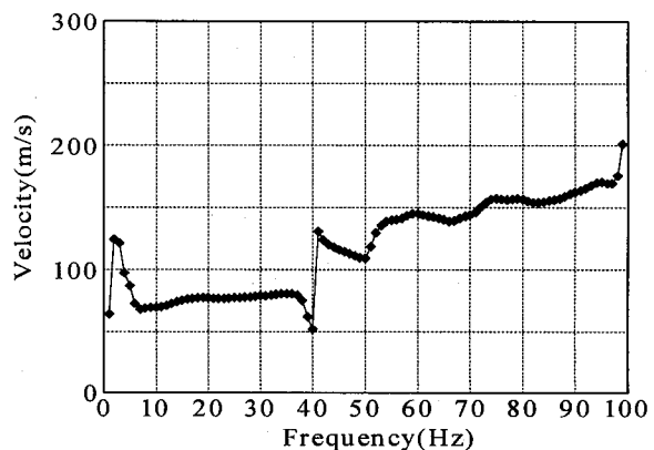
図-4 計算された位相速度 (1(m)地点)
