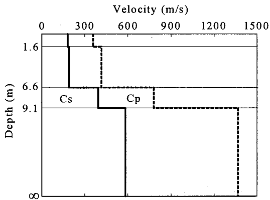
図-6 初期値地盤モデル
