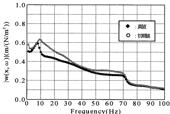
図-14 真値と初期値の鉛直変位振幅特性の比較
