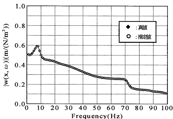
図-17 真値と推定値の鉛直変位振幅特性の比較
