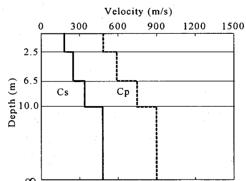
図-5 真値地盤モデル
