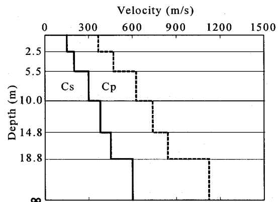
図-13 初期推定地盤モデル
