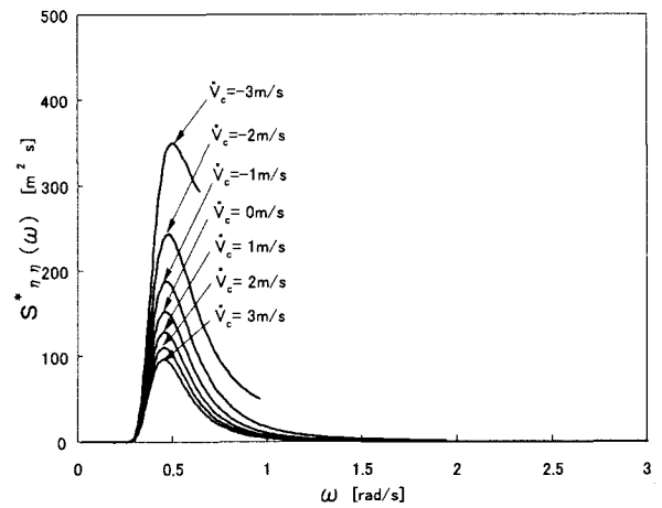
図-1 波高のパワースペクトル
