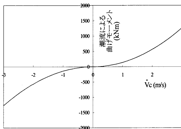
図-5 潮流による曲げモーメントと潮流の流速との関係
