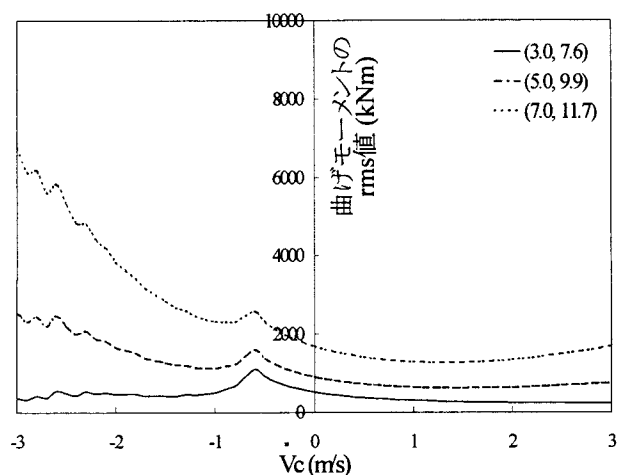
図-4 曲げモーメントのrms値と潮流の流速との関係
