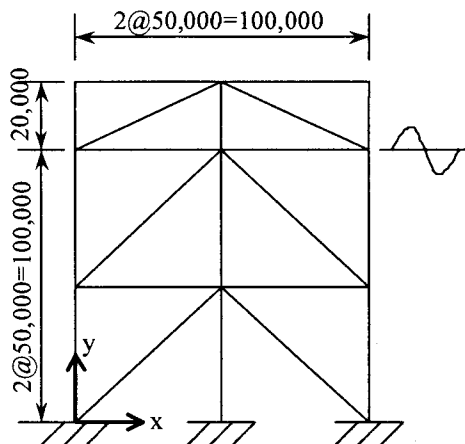
図-2 解析モデル図 (寸法の単位: mm)
