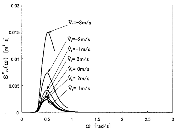
図-3 応答変位スペクトルと潮流の流速との関係
