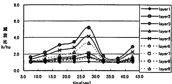
図-5(b) 各時刻、各層における正規化された減衰比(せん断剛性に重みが大さい場合、J3)
