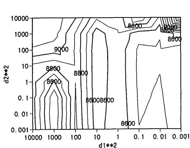
図-2 表-2におけるABICのコンター図
