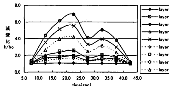
図-4(b) 各時刻、各層における正規化された減衰比(せん断剛性に重みが多い場合、J1)
