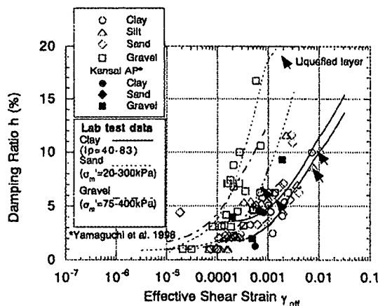
図-9 Kokusho 12) における推定地盤定数のひずみ依存性
