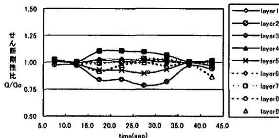
図-4(a) 各時刻、各層における正規化されたせん断剛性(せん断剛性に重みが多い場合、J1)
