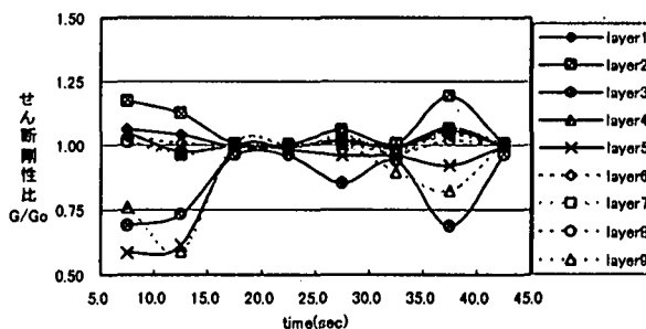
図-5(a) 各時刻、各層における正規化されたせん断剛性(せん断剛性に重みが大さい場合、J3)
