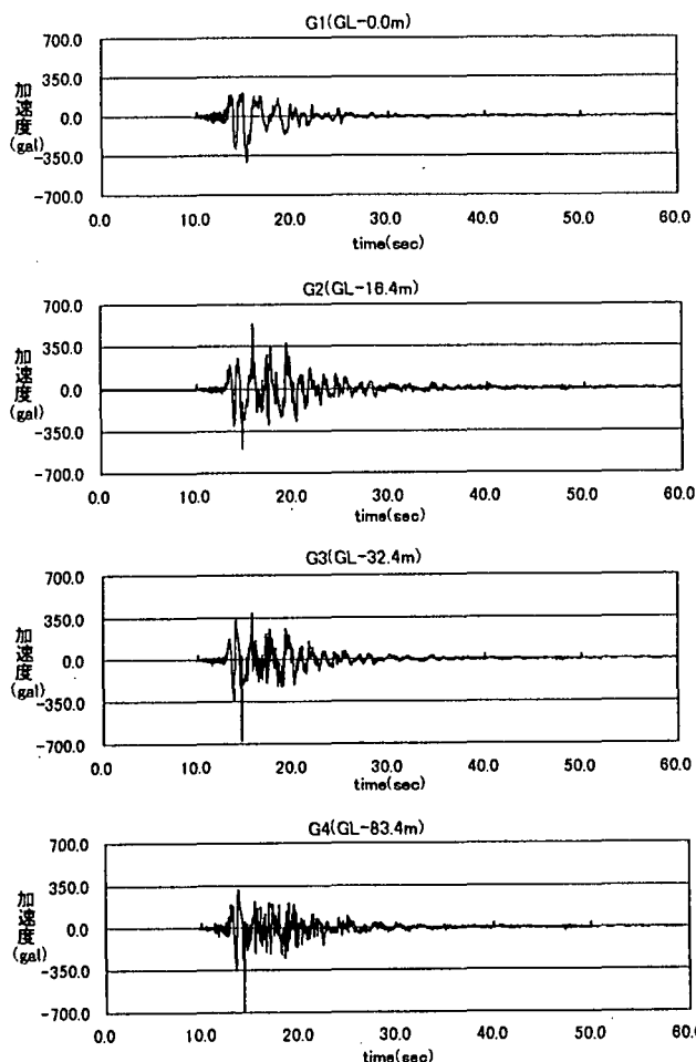
図-1 主軸方向へ変換後の加速度波形
