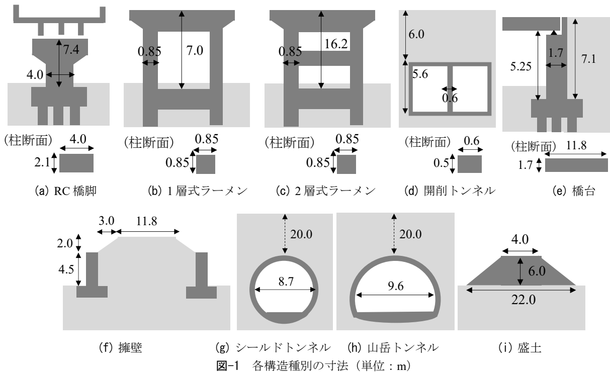
図-1 各構造種別の寸法（単位：m）
