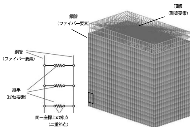
図-11 解析モデル
