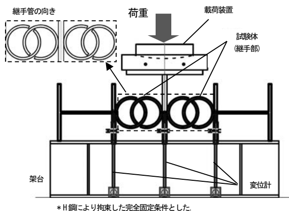
図-2 試験体概要（水平せん断試験用）
