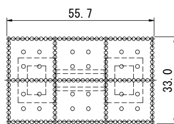
図-10 対象基礎断面図
