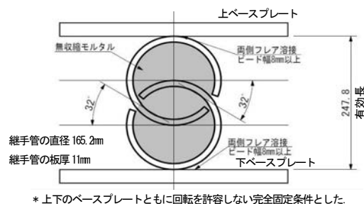
図-1 試験体概要（圧縮・引張試験用）
