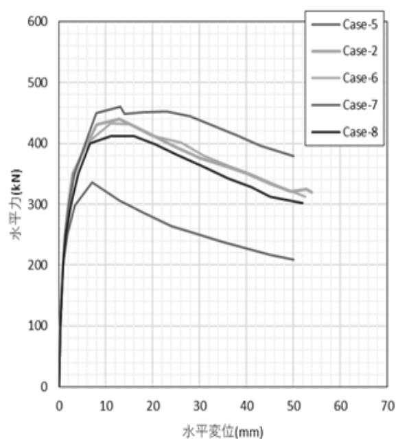
図-18 荷重—変位関係
