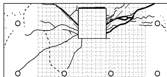
図-16 CASE2 の実験による上面ひび割れ進展 (最大荷重時 12.9mm)
