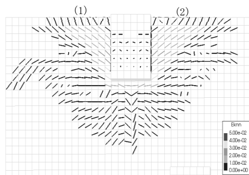
図-14 CASE2 のひび割れ進展図(15mm 進展)
