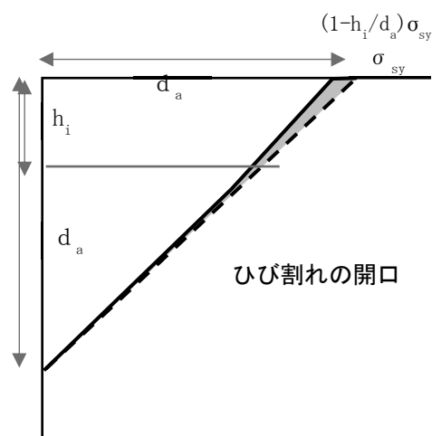
図-17 鉄筋抵抗の考え方
