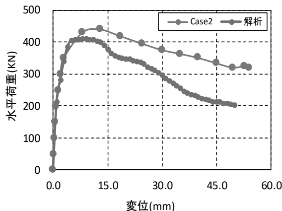
図-10 CASE2 の荷重—変位関係
