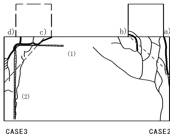
図-6 切断面のひび割れ状況
