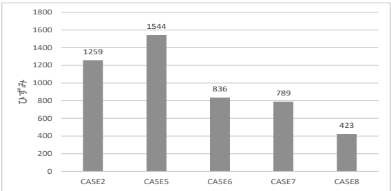
図-20 各 CASE の発生ひずみ量
