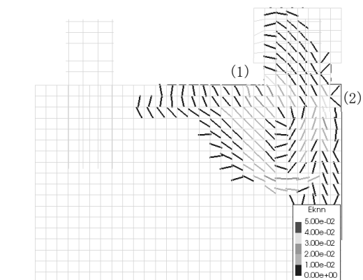
図-13 CASE2 のひび割れ進展図(10mm 進展)
