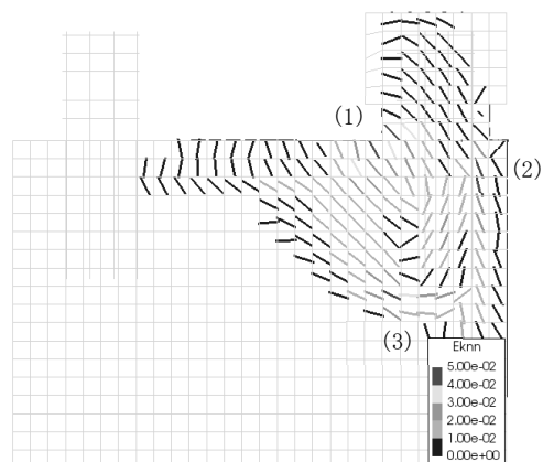
図-14 CASE2 のひび割れ進展図(15mm 進展)
