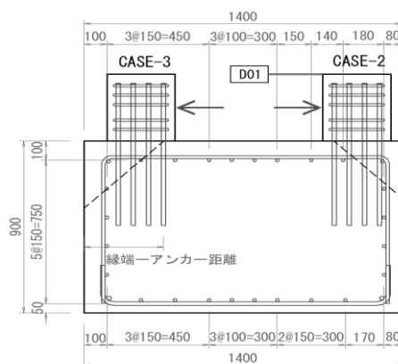
(b) 側面図
