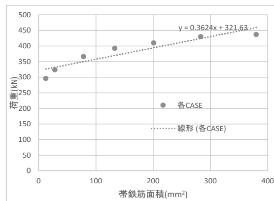
図-22 帯鉄筋量—荷重関係
