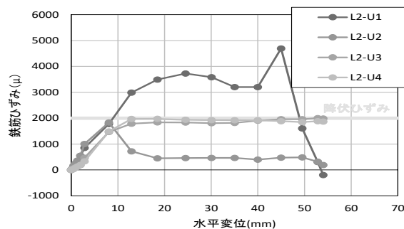
図-8 2列目計測ひずみ
