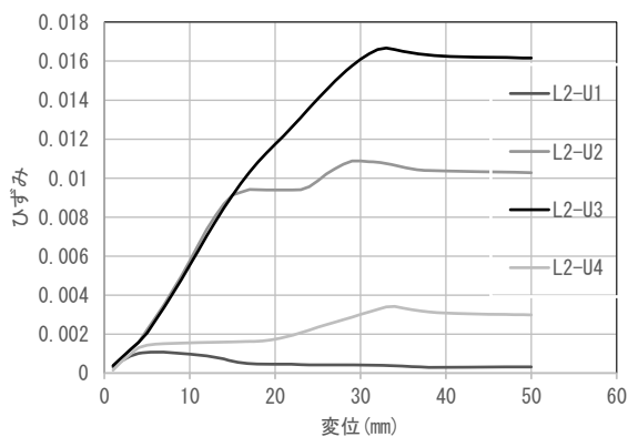
図-11 CASE2 の荷重—ひずみ（2列目）
