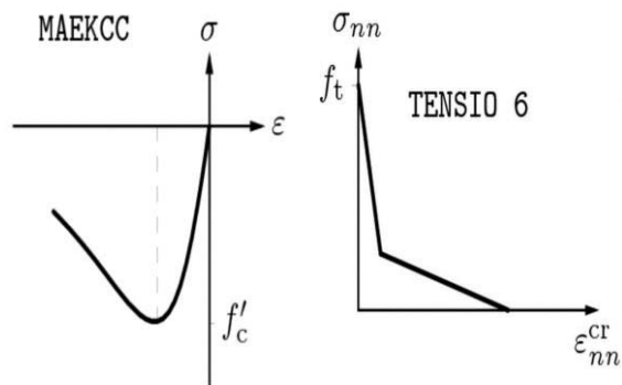
図-3 圧縮および引張応力ひずみモデル
