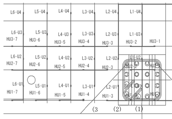
図-7 計測ひずみ点
