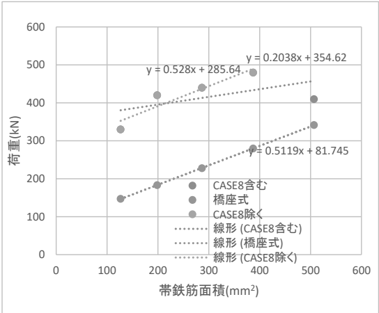
図-19 帯鉄筋量－荷重関係
