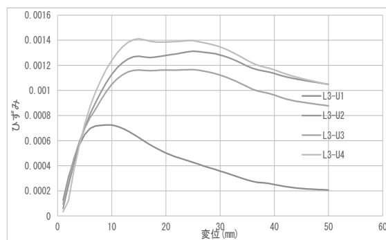
図-12 CASE2 の荷重—ひずみ（3列）
