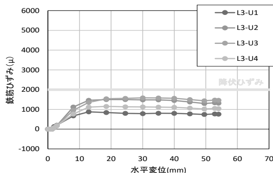
図-9 3列目計測ひずみ
