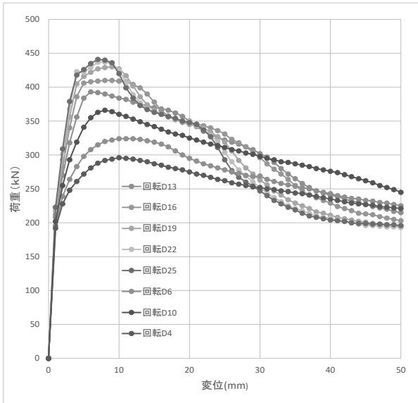
図-21 各 CASE の荷重－変位関係
