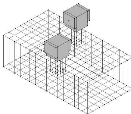
図-2 供試体モデル
