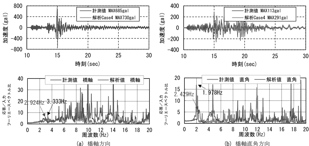
図-16 Case4:加速度応答時刻歴（上段）とフーリエスペクトル比（下段）
