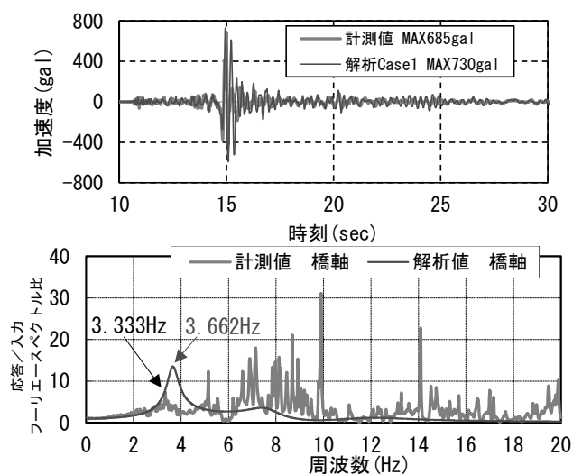
(a) 橋軸方向
