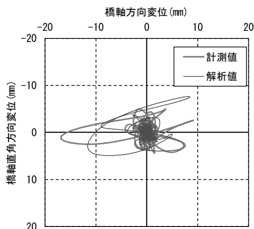
(c) 橋軸-橋軸直角方向の関係
