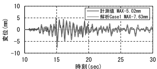
(b) 橋軸直角方向時刻歴
