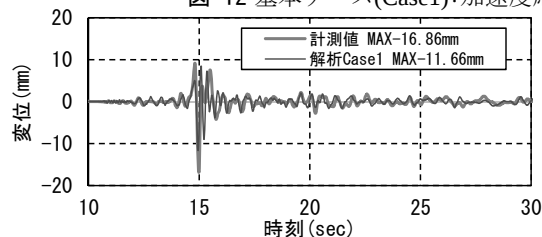
(a) 橋軸方向時刻歴
