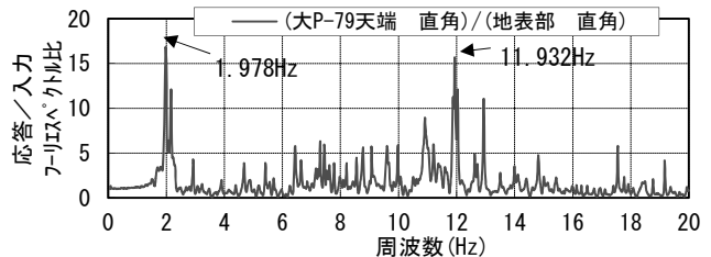
(b) 橋軸直角方向
