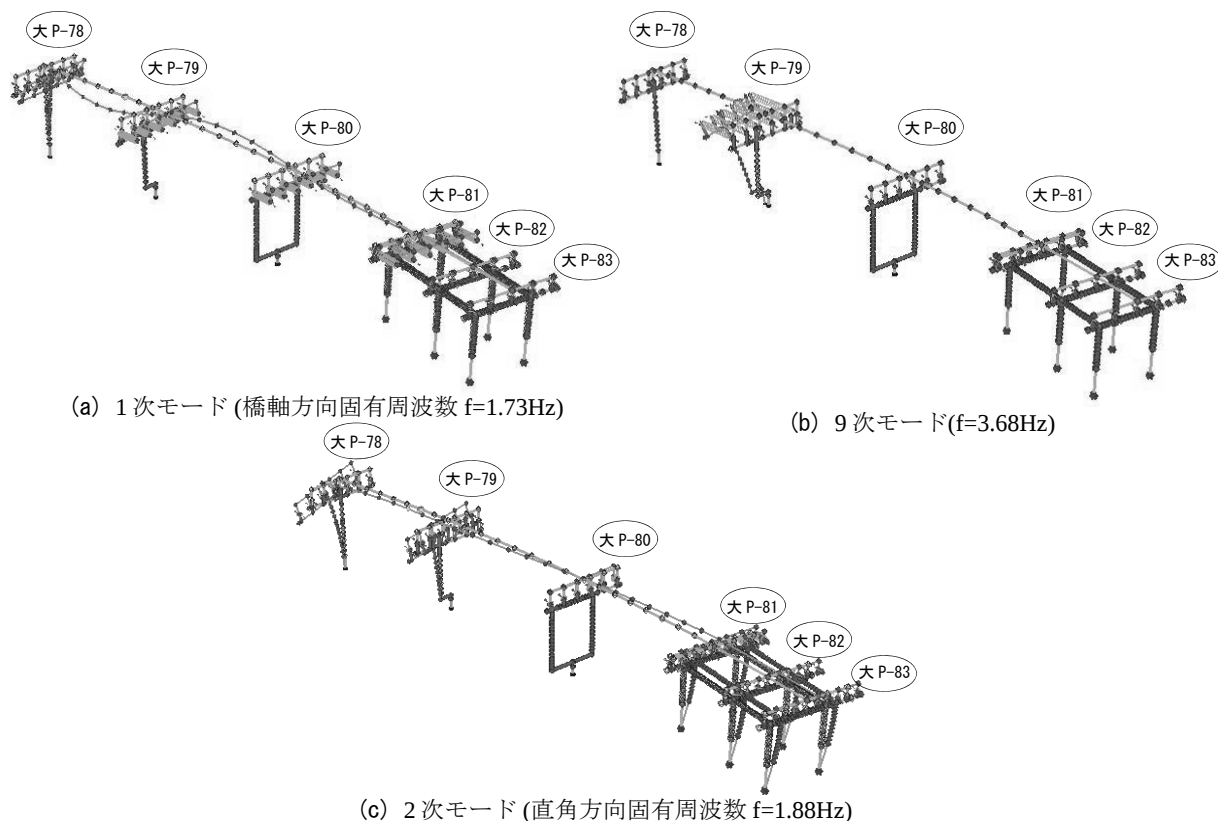
図-10 主要振動モード図
