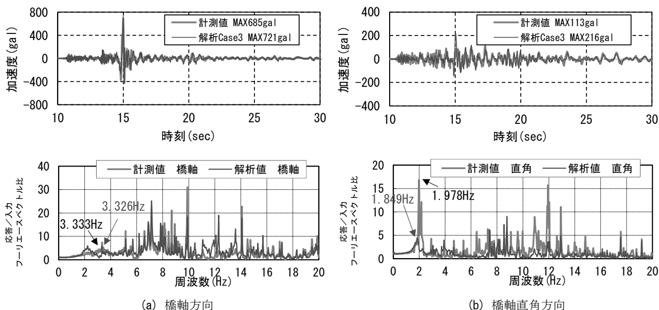
図-15 Case3:加速度応答時刻歴（上段）とフーリエスペクトル比（下段）
