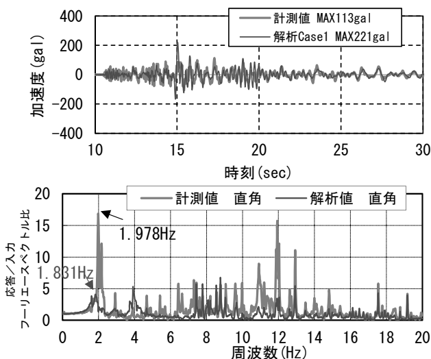
(b) 橋軸直角方向
