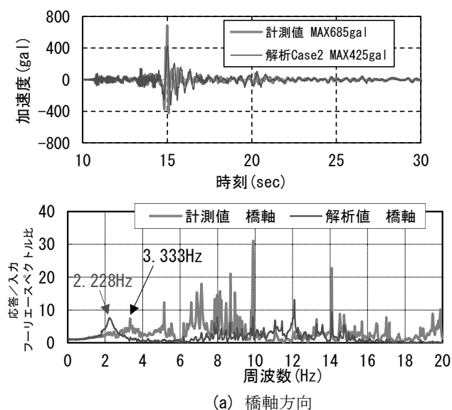
図-14 Case2: 加速度応答時刻歴（上段）とフーリエスペクトル比（下段）
