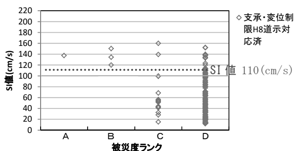
図-7 SI値と被災度の関係
