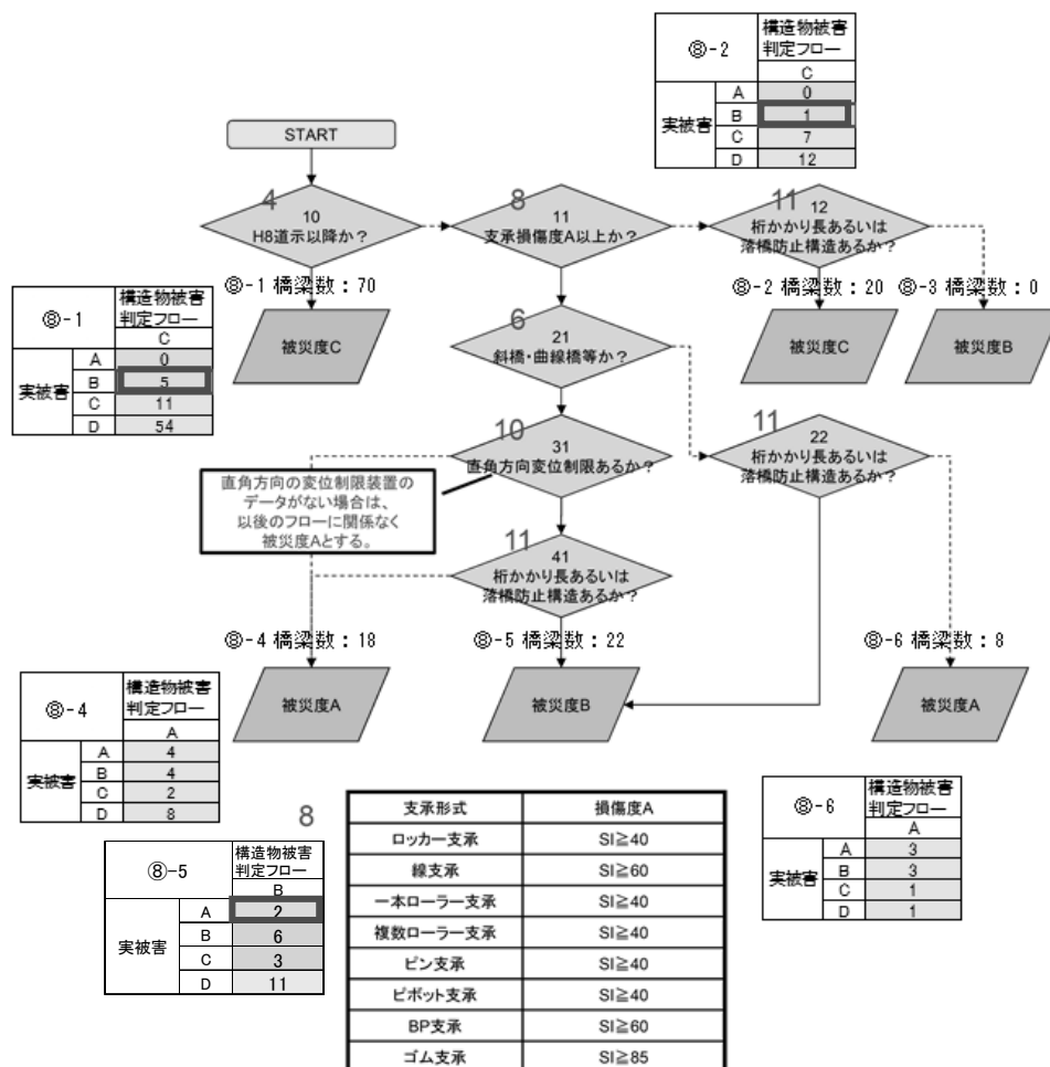
図-4 危険側の推定結果箇所（B-3 支承・落橋防止）
