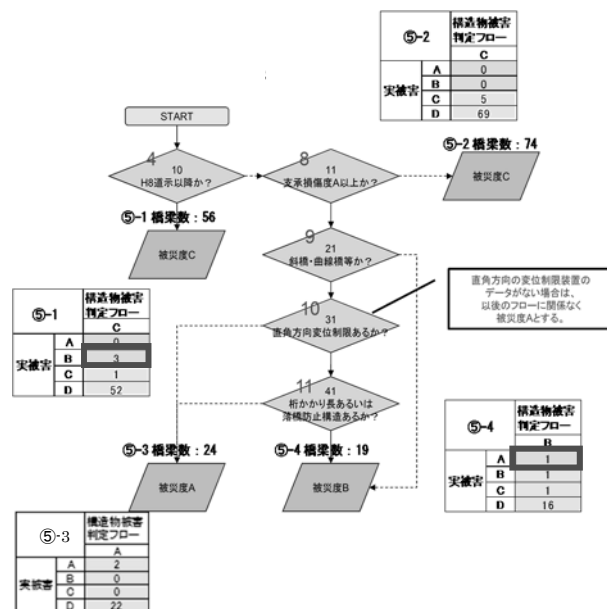
図-6 危険側の推定結果箇所（A-1 端部支承・落橋防止）
