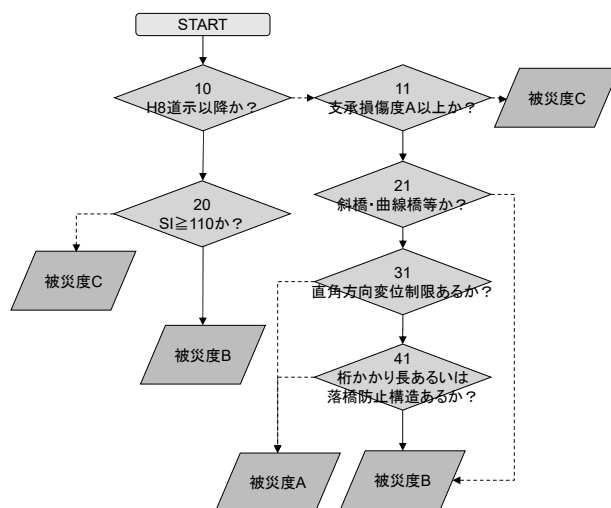
図-8 A-1 端部支承・落橋防止（改良後）
