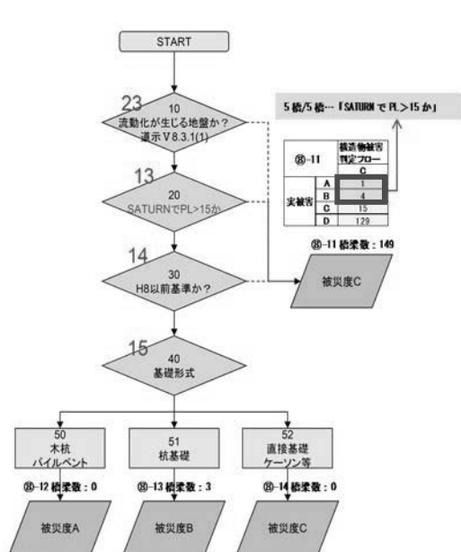
図-5 危険側推定結果箇所（B-5 橋梁基礎側方流動の評価）
