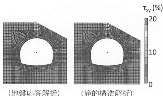
図 11 セン断ひずみ分布の比較 (ケース 3)
