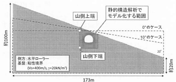
図3 地盤応答解析の概念図
