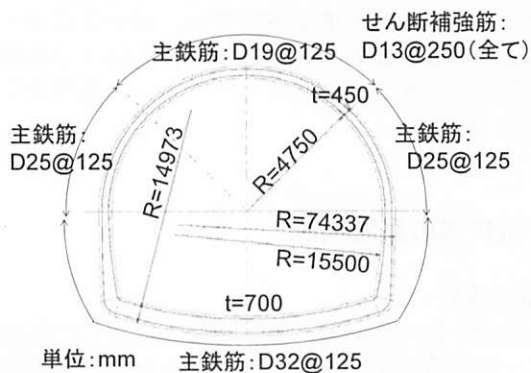
図 7 常時設計による決定断面
