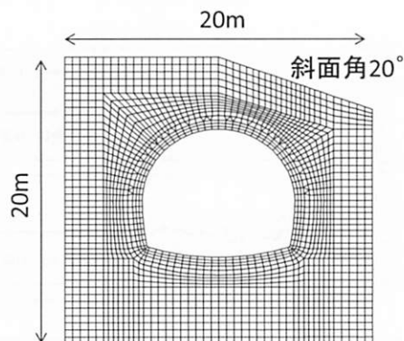
(b) ケース 3 (斜面角度 20°)
