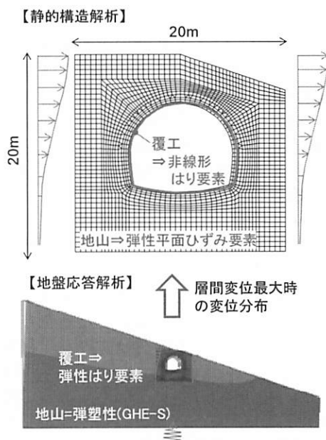
図1 適用するFEM応答変位法の概念図
