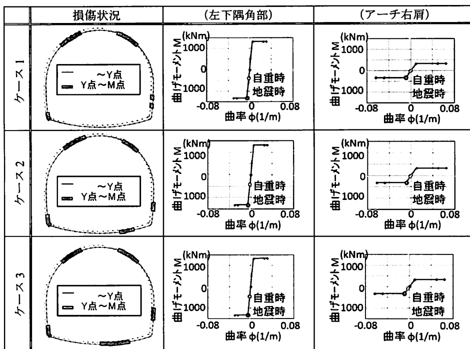
図10 覆工の曲げ損傷の進展
