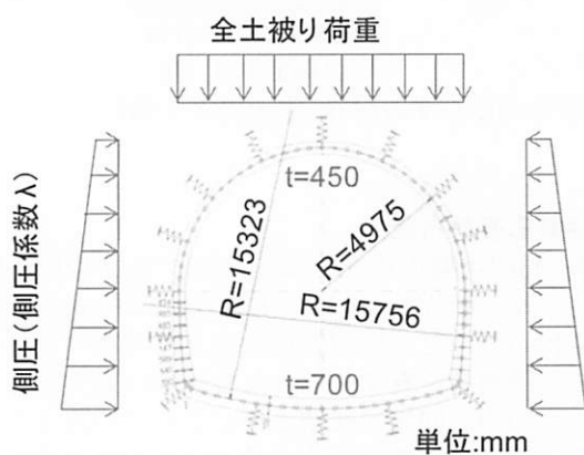
図 6 常時設計で考慮した荷重
