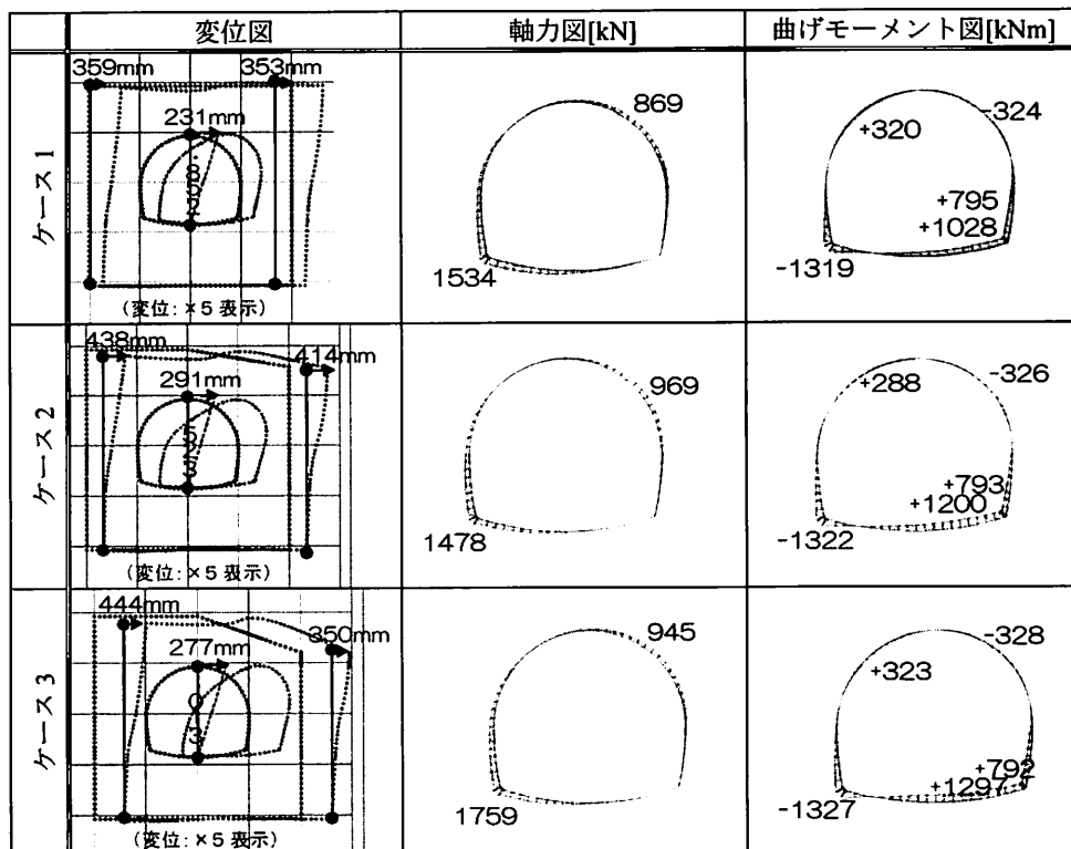
図9 トンネルの応答 (変形, 断面力)
