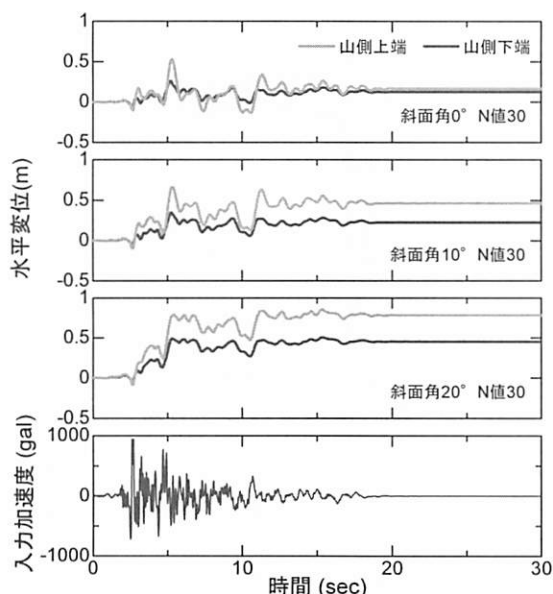
図4 周辺地盤上下端の変位時刻歴
