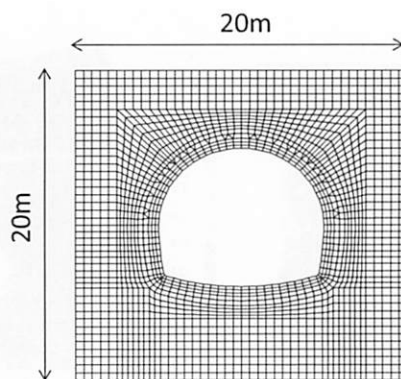
(a) ケース 1 (整形地盤)
