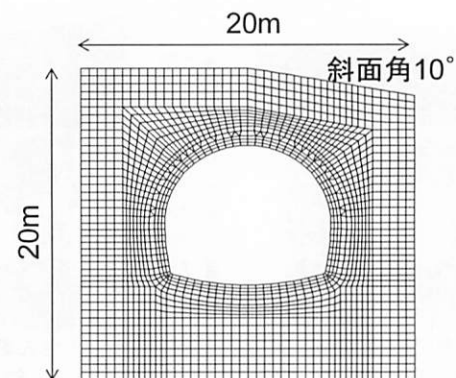
(b) ケース 2 (斜面角度 10°)
