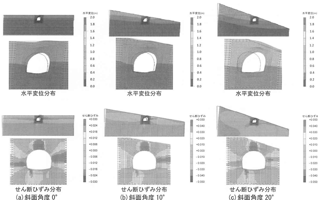
図5 上下端相対変位最大時の周辺地盤の変位およびせん断ひずみ分布(表示倍率5倍)
