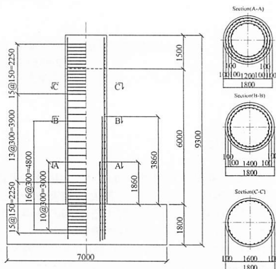
圖-4 C1-2橋脚模型
