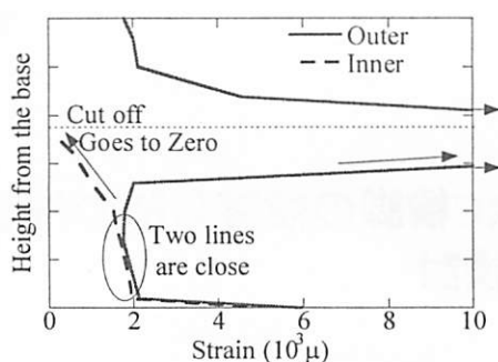
図-1 段落し位置周辺の軸方向鉄筋ひずみ
