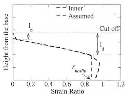
図-2 段落し位置周辺の軸方向鉄筋ひずみ比
