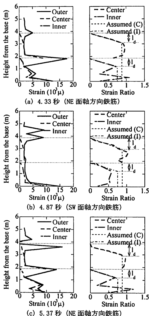
図-5 引張側軸方向鉄筋ひずみ（左：軸方向鉄筋ひずみ，右：軸方向鉄筋ひずみ比）
