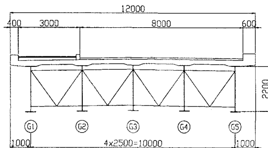
図-3 断面図
