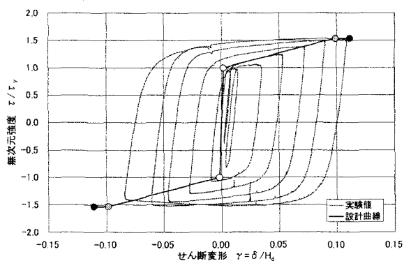
図-14 実験値と設計曲線の比較
