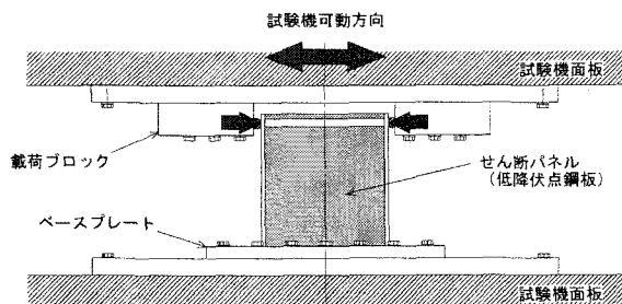
図-13 正負交番载荷試験概要
