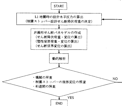
図-5 制震ストッパー設計フロー
