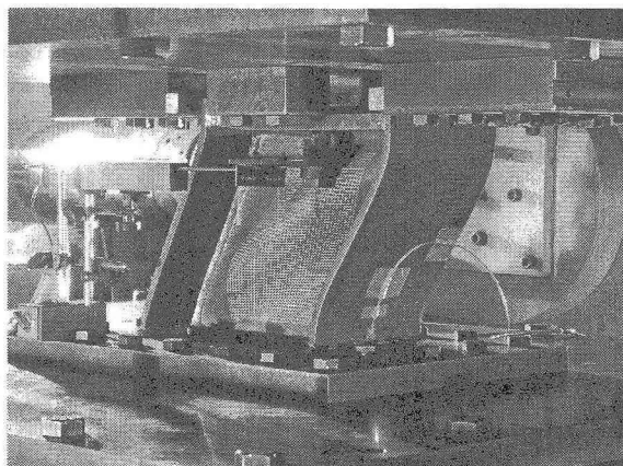
写真-1 終局状態でのウェブの変形状況
