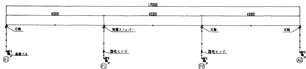
図-4 解析モデル(3径間連続I桁橋)
