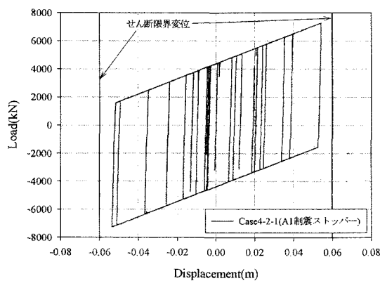
図-7 制震ストッパー履歴曲線(2径間連続I桁橋)
