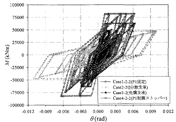
図-8 M-θ関係(2径間連続I桁橋)
