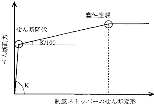
図-2 制震ストッパーの履歴特性
