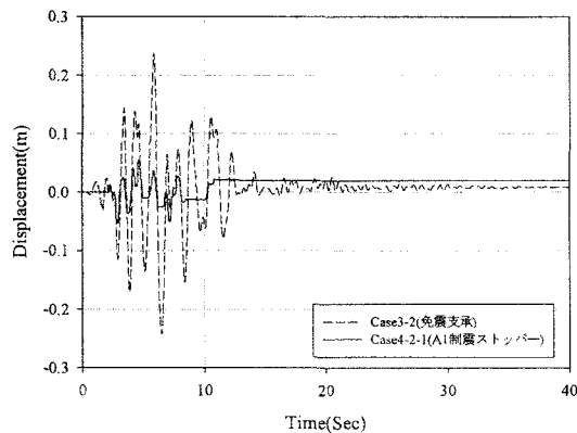
図-6 時刻歴応答変位(2径間連続I桁橋)
