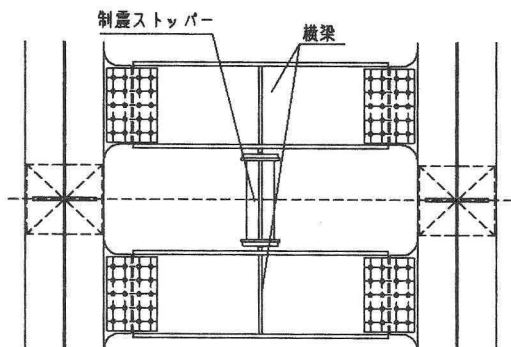
図-9 制震ストッパーの設置例
