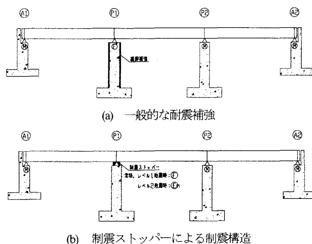
図-1 制震ストッパー設置例
