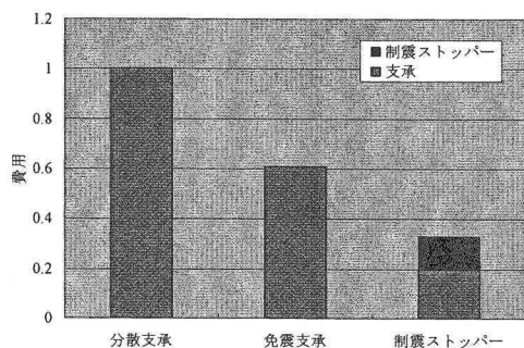
図-10 支承形式による経済性の比較(2径間連続I桁橋)
