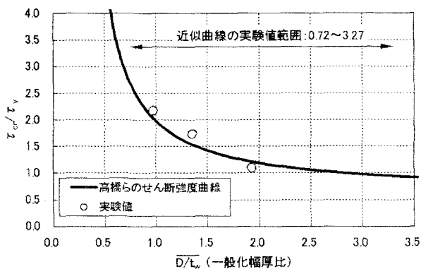
図-12 実験値と評価式のせん断座屈耐力の比較
