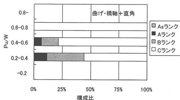
図-8 P_u/W の損傷度の構成比(曲げ損傷)
