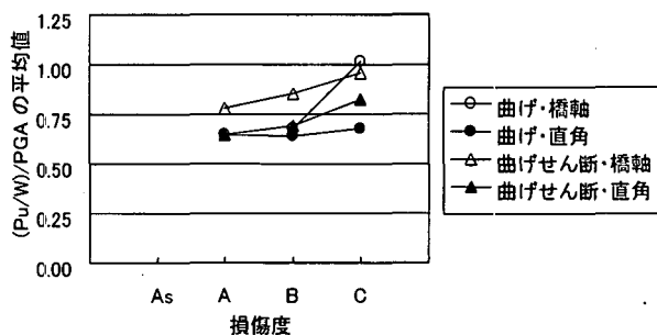
図-7 損傷度別の (P_u/W)/PGA の平均値(曲げ, 曲げせん断損傷)
