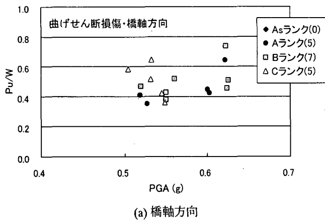
図-5 損傷度別の P_u/W の平均値(曲げ, 曲げせん断損傷)
