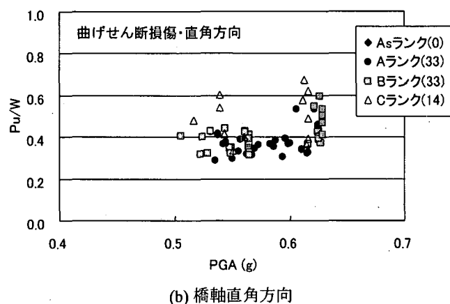
図-4 PGAと P_u/W の関係(曲げせん断損傷)
