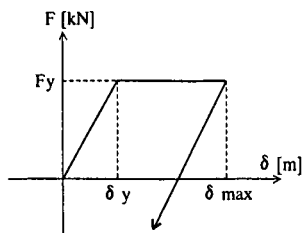
図-2 非線形履歴特性
