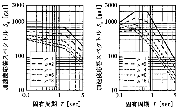
(a) タイプ I の地震動
