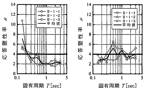
(a) エネルギー一定則 (b) 提案式 図-10 非線形動的解析による応答塑性率 (タイプⅡの地震動, Ⅰ種地盤)
