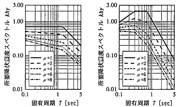
(a) タイプ I の地震動
