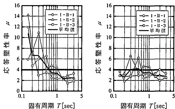
(a) エネルギー一定則 (b) 提案式 図-9 非線形動的解析による応答塑性率 (タイプⅠの地震動, Ⅱ種地盤)
