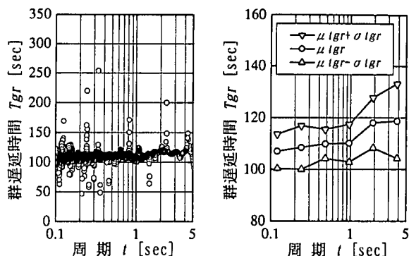
図-3 尼崎高架橋 HA 成分の群遅延時間
