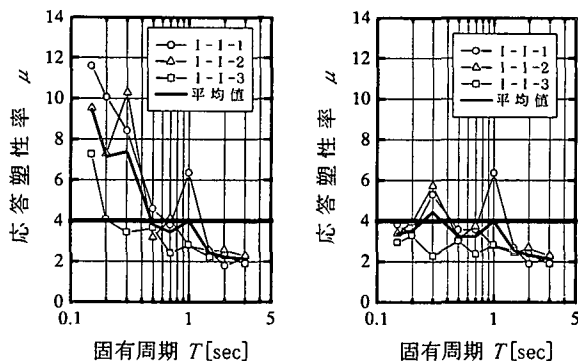
(a) エネルギー一定則 (b) 提案式 図-8 非線形動的解析による応答塑性率 (タイプⅠの地震動, Ⅰ種地盤)
