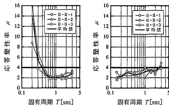
(a) エネルギー一定則 (b) 提案式 図-11 非線形動的解析による応答塑性率 (タイプⅡの地震動, Ⅱ種地盤)
