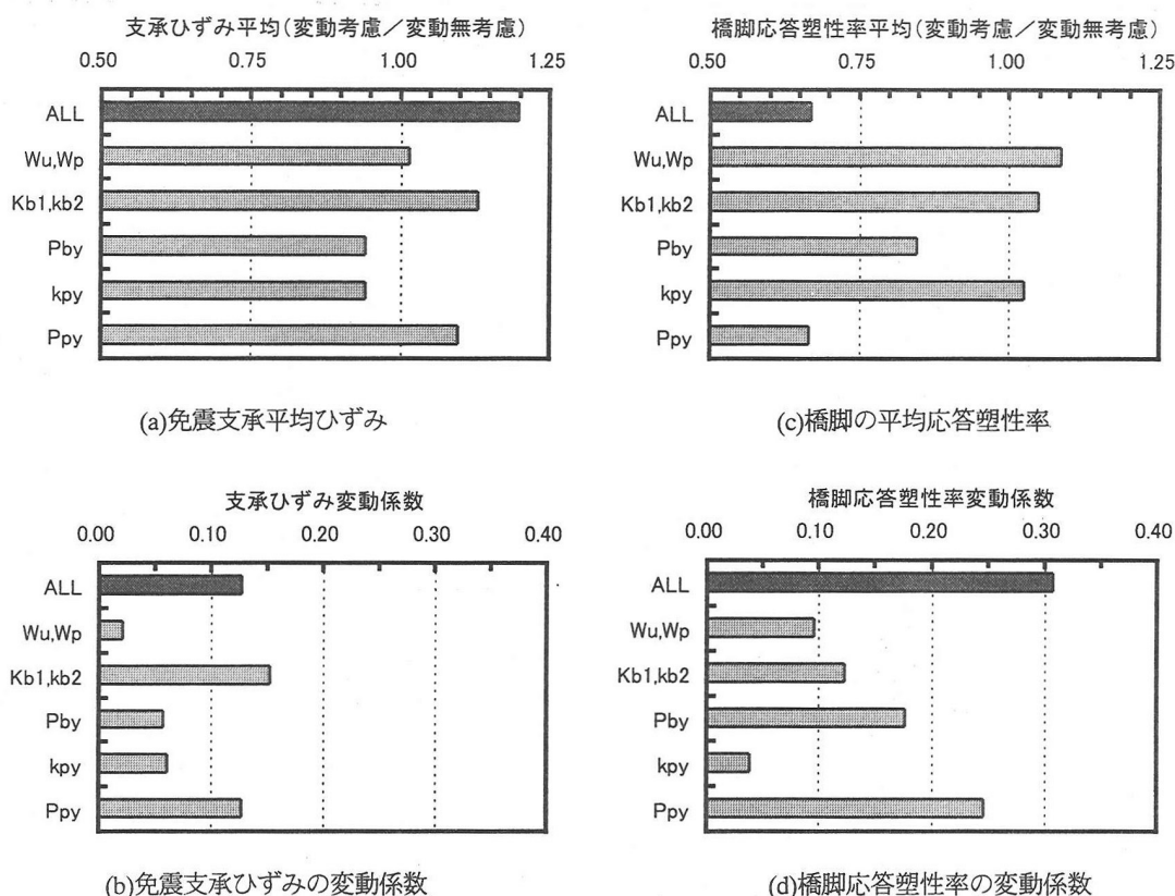
図-14 変動要因が免震支承および橋脚の地震応答に及ぼす影響に関する感度分析 (LRB の場合)
