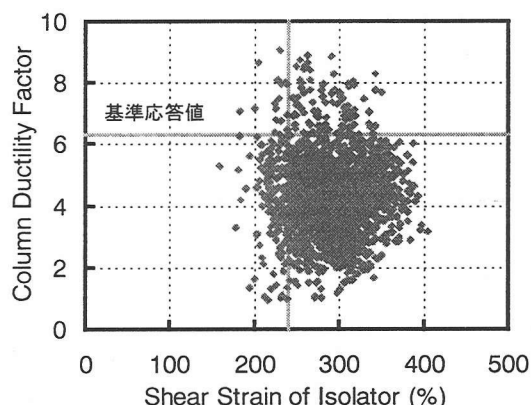
図-13 橋脚塑性率と支保ひずみとの関係 (LRB)
