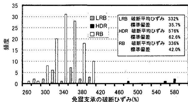
図-7 免震支承の破断ひずみ分布特性
