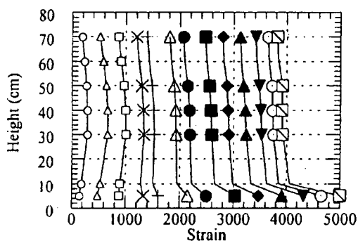
図-9 芯材の高さ方向のひずみ分布
