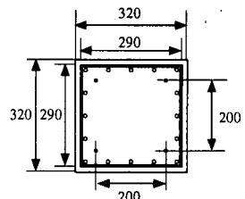
(d) No. 4 供試体
