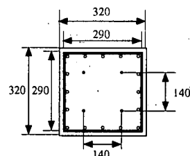
(b) No. 2 供試体
