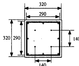
(c) No. 3 供試体
