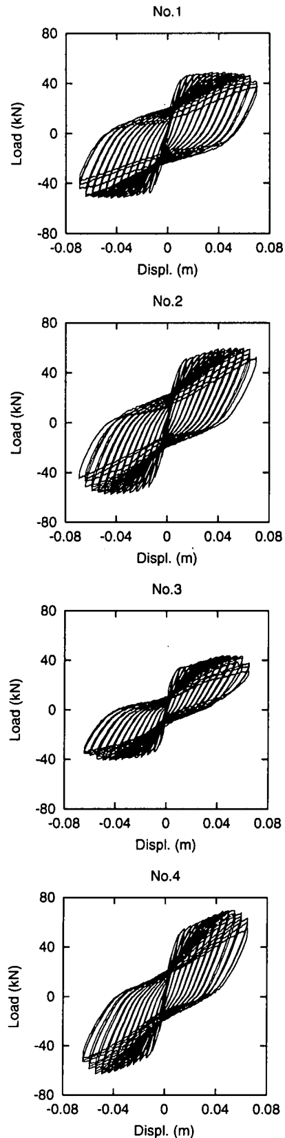
図-5 実験による荷重-変位関係
