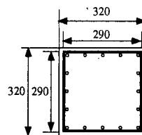
(a) No. 1 供試体
