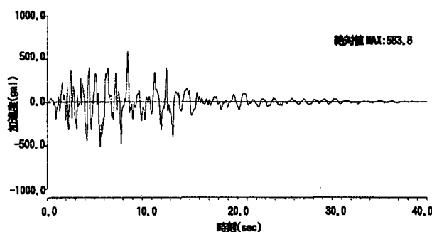
図-10 引き戻し前の地表面波形
