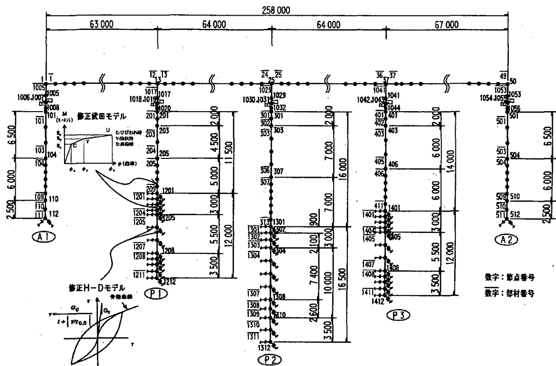
図-9 連成解析モデル
