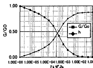
図-7 G/G_0 ・ \gamma ・ h ・ \gamma の関係
