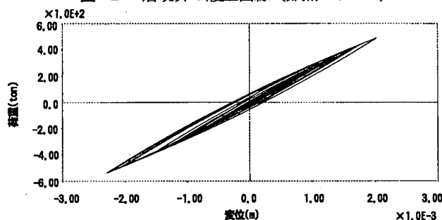
図-24 層境界の履歴曲線（節点 No. 1308）
