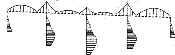
図-26 最大曲げモーメント図
