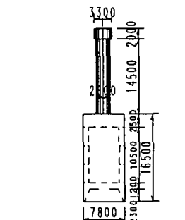
図-2 P2橋脚側面図
