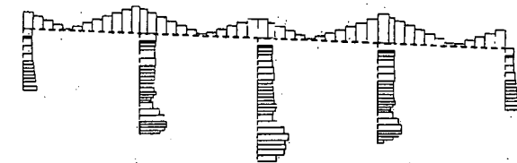
図-27 最大せん断力図
