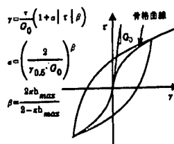
図-8 修正R-Oモデル
