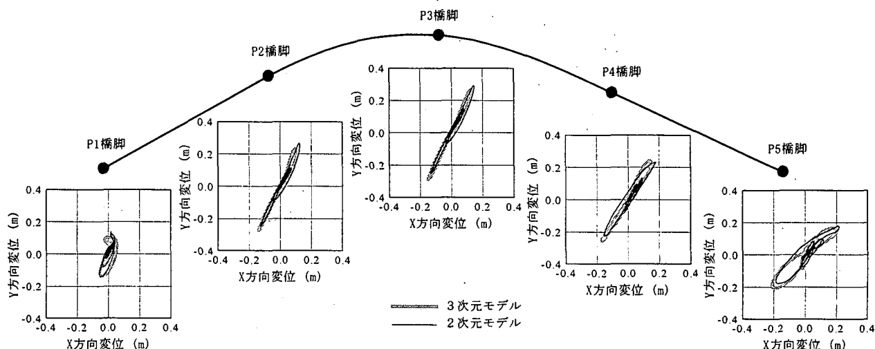
図-5 各橋脚の上部構造慣性力作用位置の最大応答水平変位（入力方向 60°）
