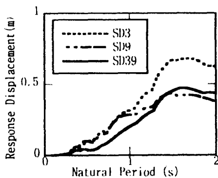
(b) 相対変位応答スペクトル
