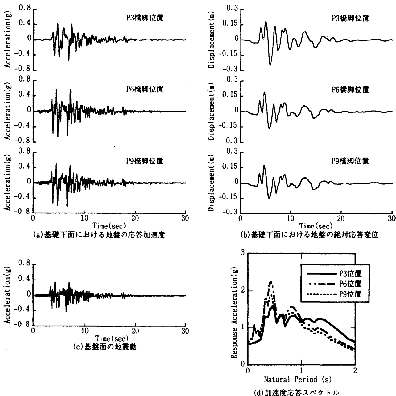
図8 表層地盤の動的応答（神戸海洋気象台記録を作用させた場合）
