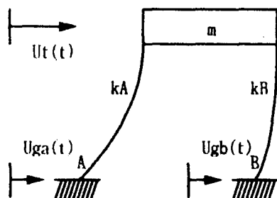
図 - 15 マルチサポート応答スペクトル
