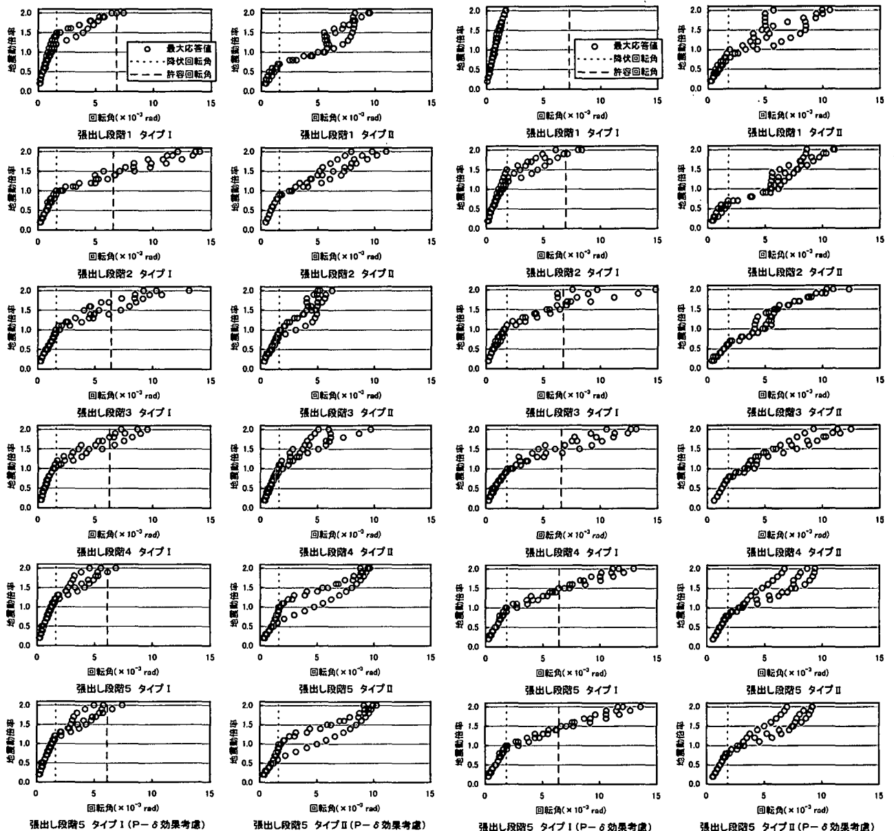
図-11 橋脚下端塑性ヒンジ回転角 (H=30m 橋軸方向)
