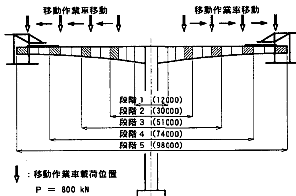
図-3 設定した張出し段階
