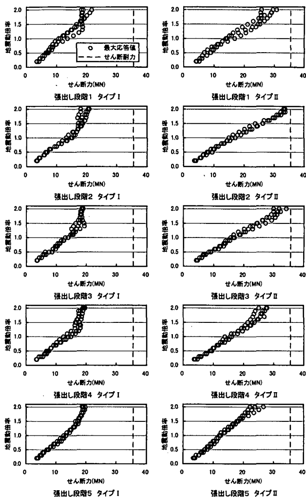
図-18 橋脚下端せん断力 (H=60m 直角方向)
