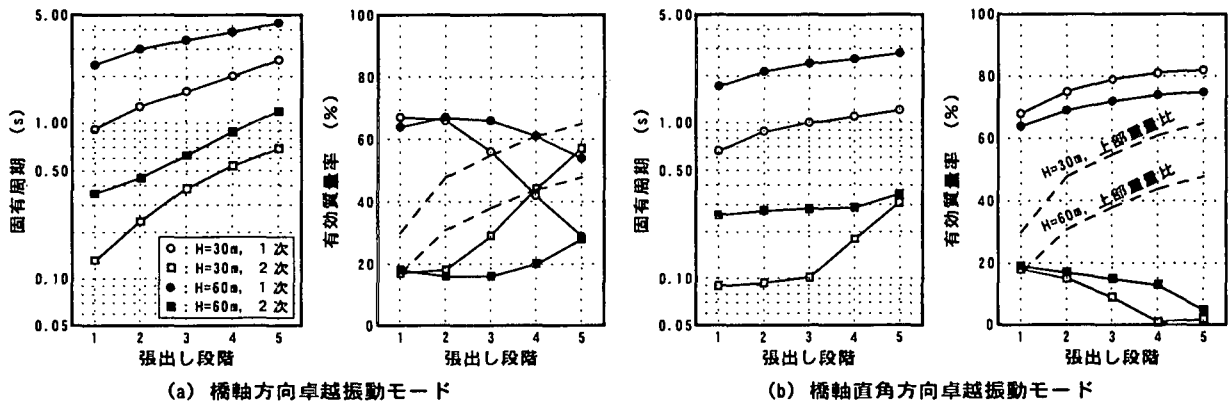
図-10 張出し施工時の固有周期および有効質量率
