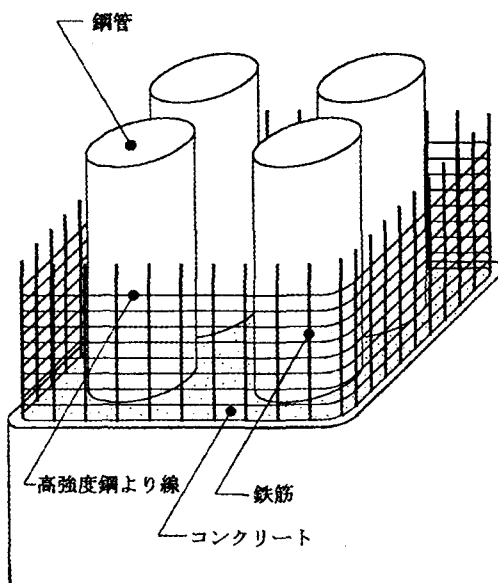
図-1 鋼管・コンクリート複合構造橋脚概念図
