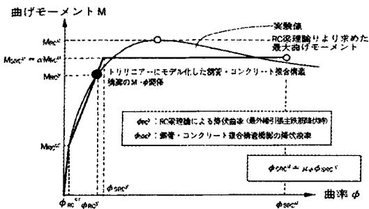
図-5 本構造の橋脚断面のモーメント-曲率関係
