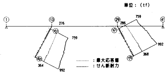
図-6 橋脚のせん断力 (橋軸直角方向)
