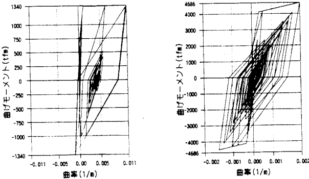
P1橋脚上部一橋軸方向 P1橋脚下部一橋軸直角方向
