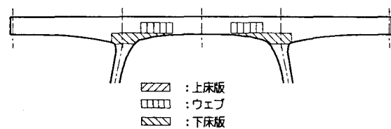
図-11 上部工鉄筋補強位置
