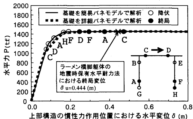
図-7 全体系の水平力-水平変位関係
