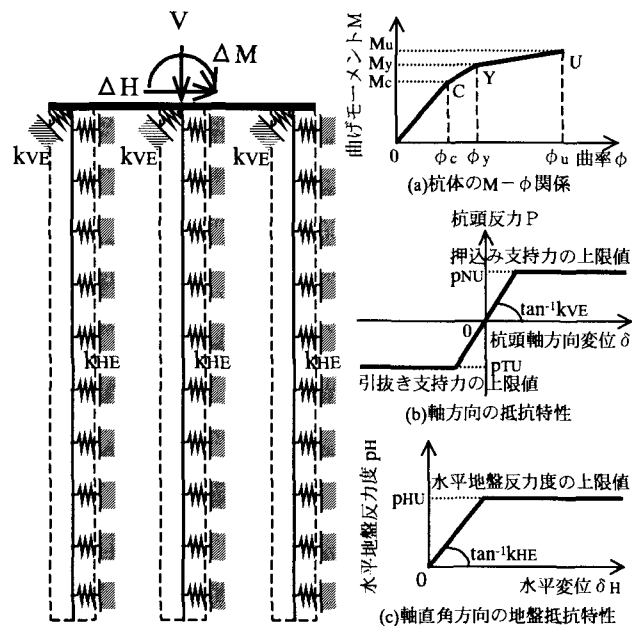
図-2 杭基礎の解析モデル
