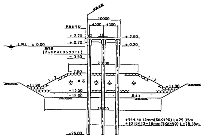
図-4 神戸港直杭式棧橋の標準断面
