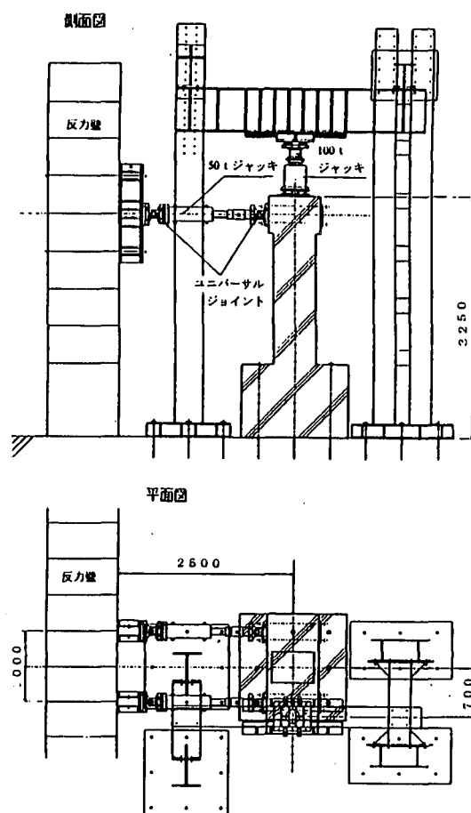
図-3 载荷装置
