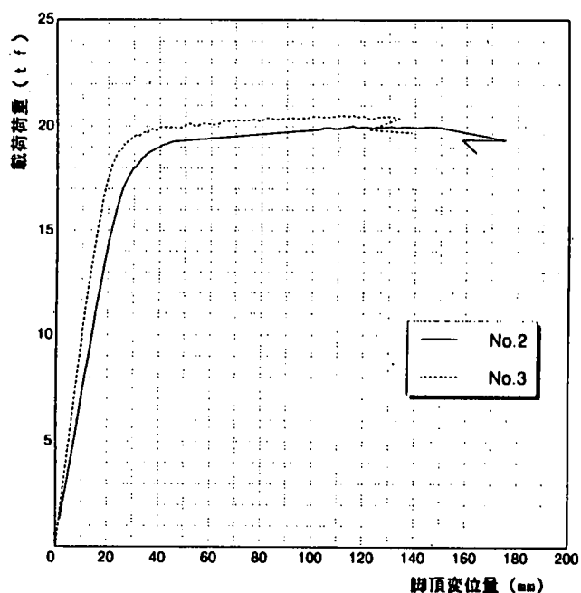
図-8 実験終了後の供試体の耐力
