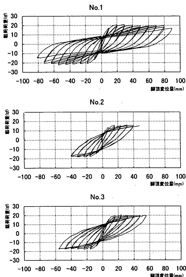
図-4 P— \delta 曲線
