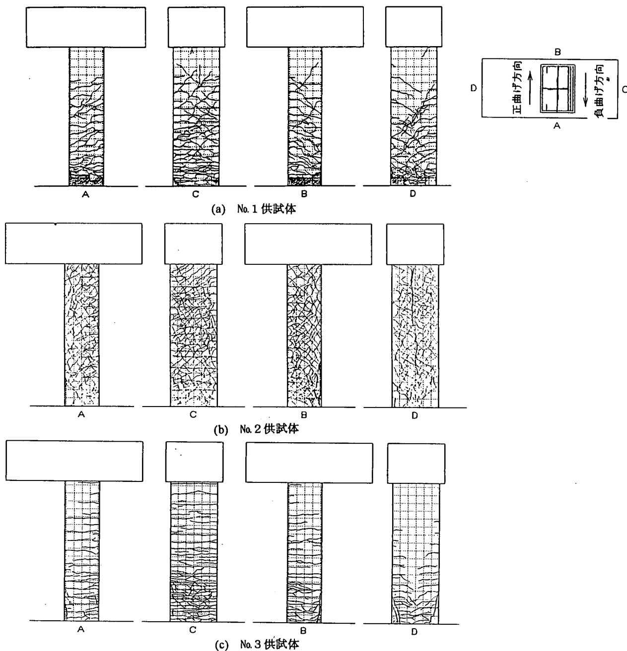
図-7 ひびわれ図
