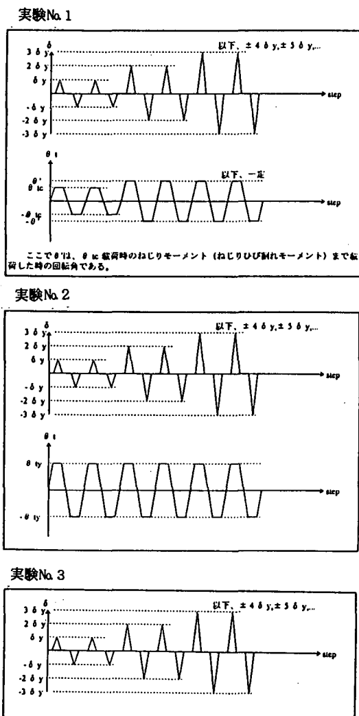
図-2 载荷ステップ
